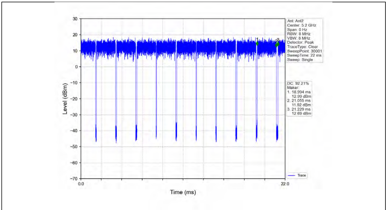
802.11a_HCH_5240MHz_Ant2_NTNV
