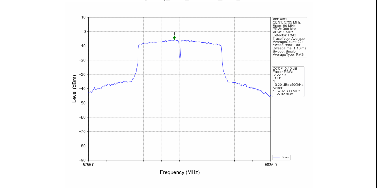
802.11n(HT40)_HCH_5795MHz_MIMO_NTNV
