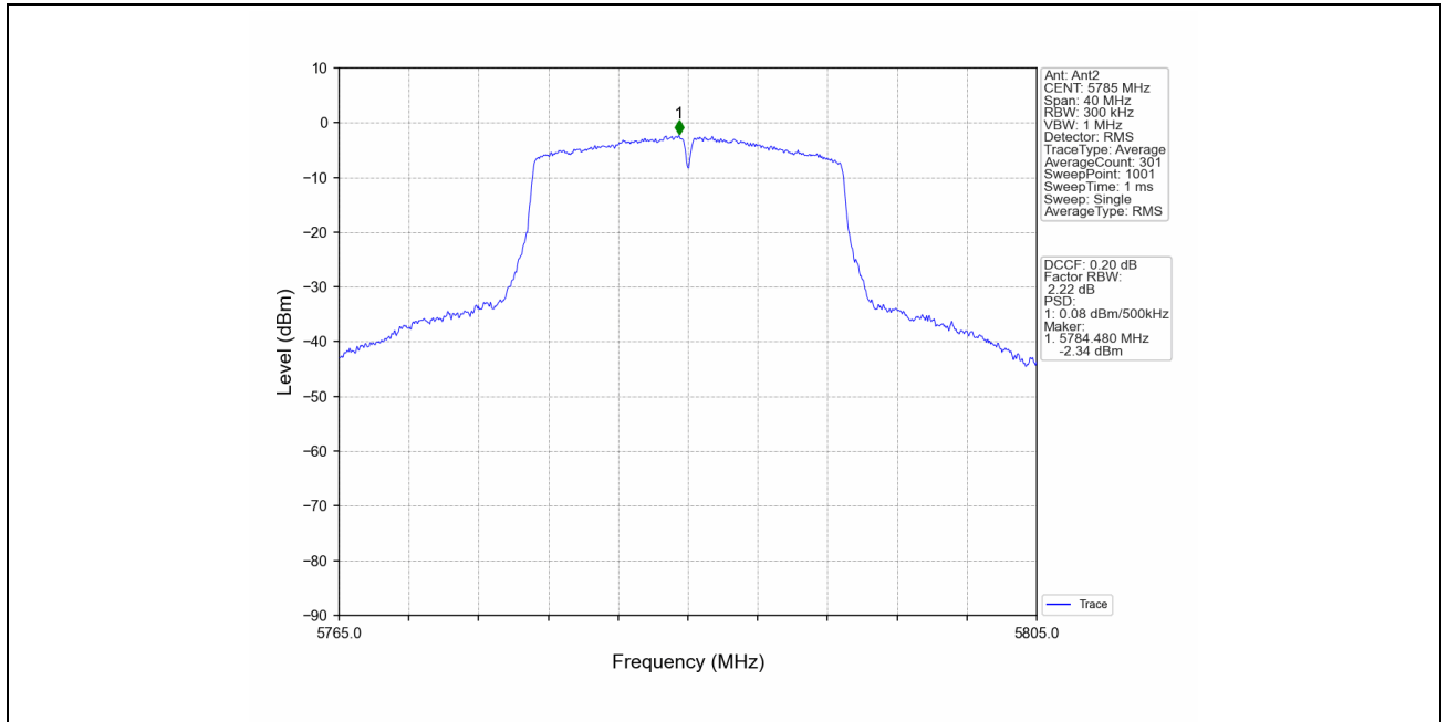
802.11n(HT20)_MCH_5785MHz_MIMO_NTNV
