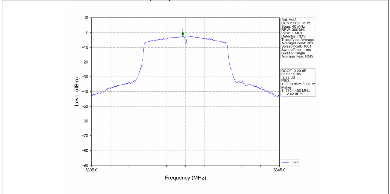
802.11n(HT20)_HCH_5825MHz_MIMO_NTNV
