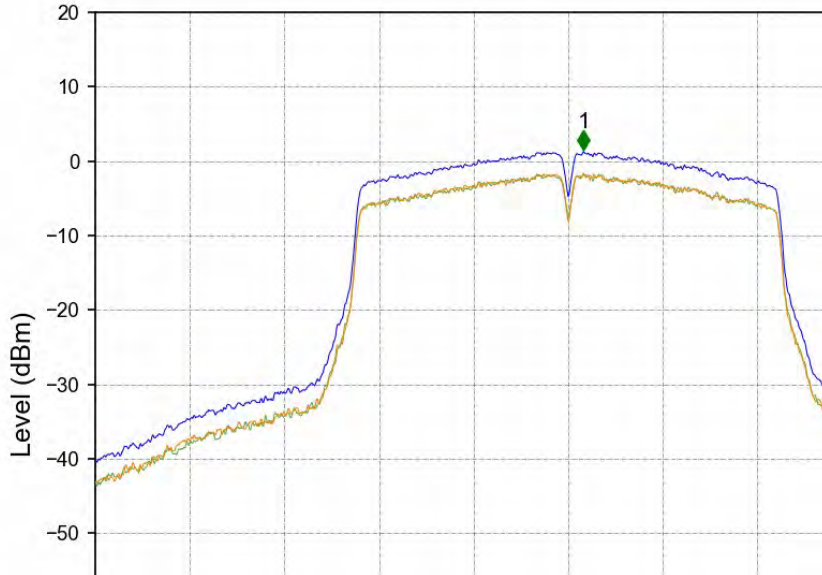
802.11n(HT20)_MCH_5785MHz_Ant1_NTNV
