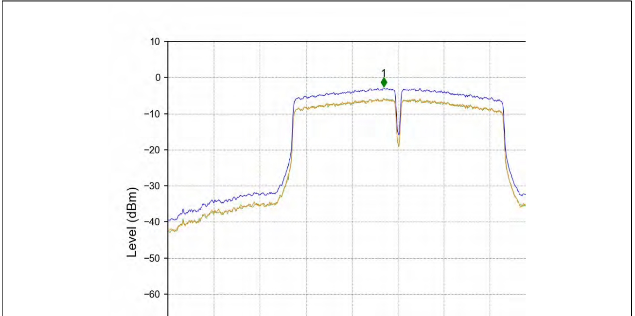
802.11ac(VHT20) LCH_5745MHz Ant1 NTNv
