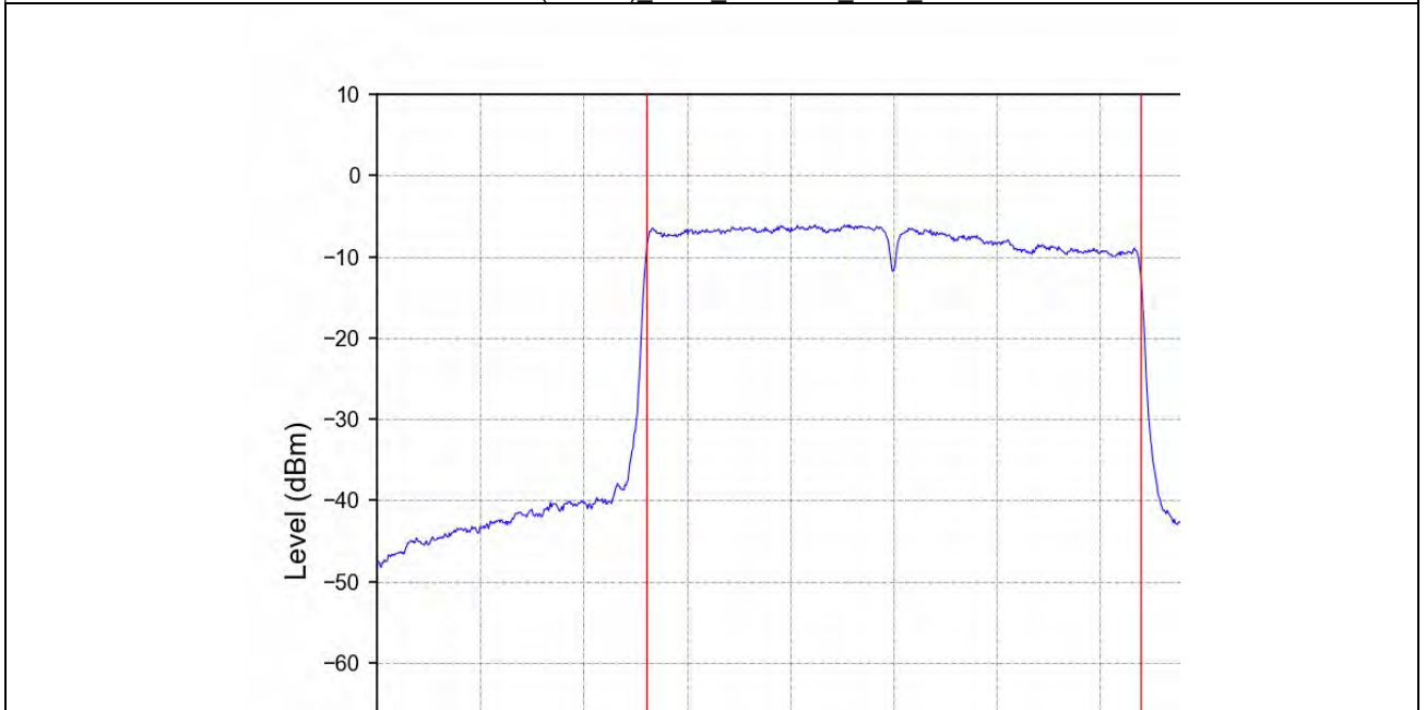
802.11ac(VHT80) MCH 5775MHz Ant2 NTVN
