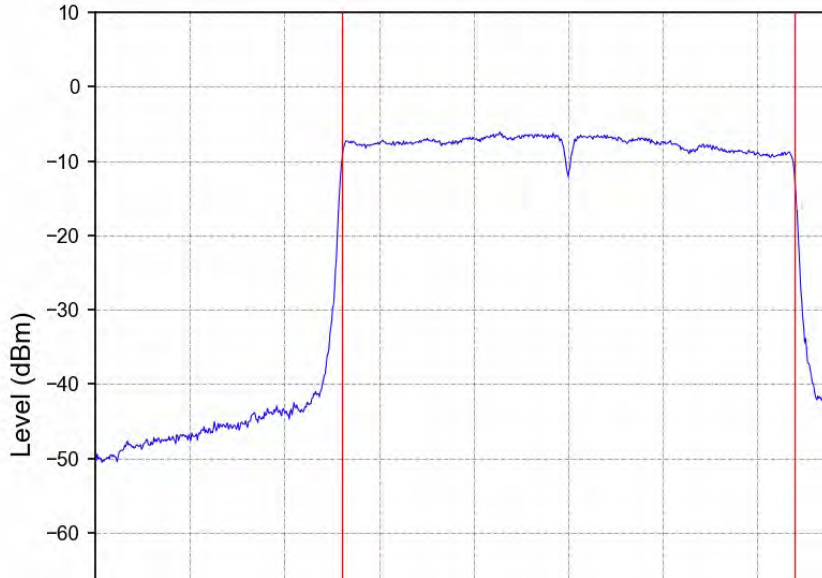
802.11ac(VHT80) MCH 5290MHz Ant2 NTNv
