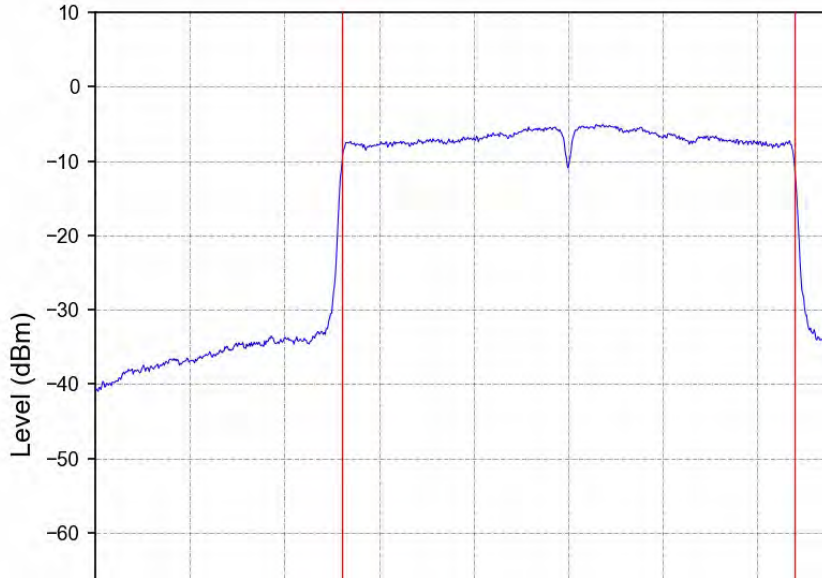
802.11ac(VHT80) HCH 5610MHz Ant2 NTV
