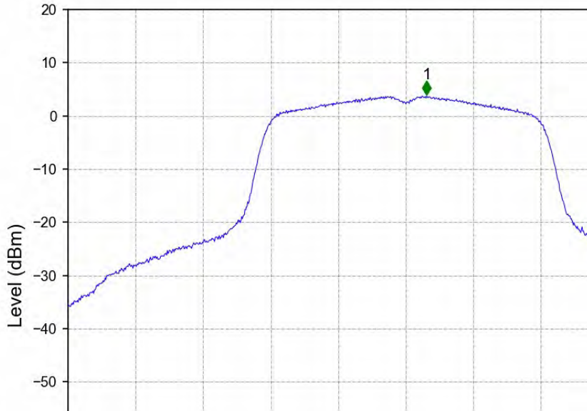
802.11a_LCH_5500MHz_Ant2_NTNV
