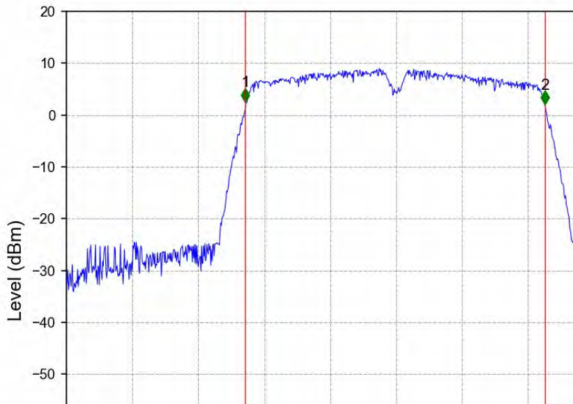
802.11ac(VHT40) HCH_5230MHz_Ant1_NTNV
