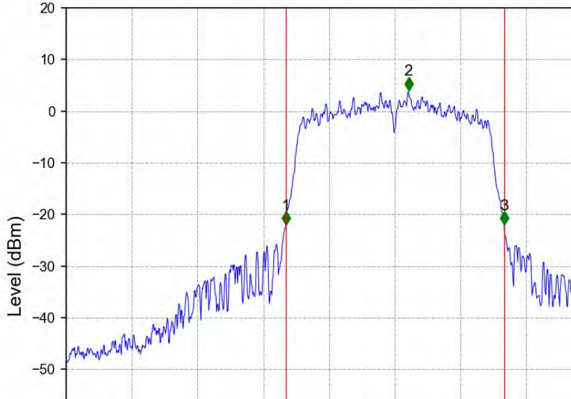
802.11n(HT20)_MCH_5200MHz_Ant2_NTNV
