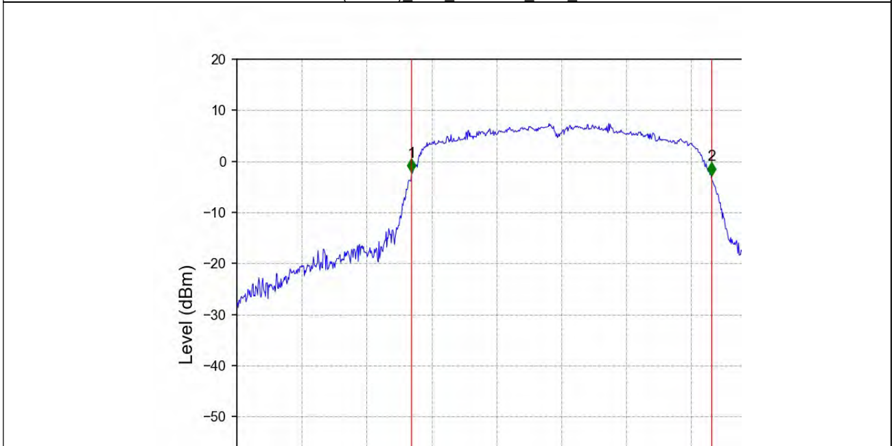
802.11ac(VHT20) MCH_5580MHz_Ant1_NTNV
