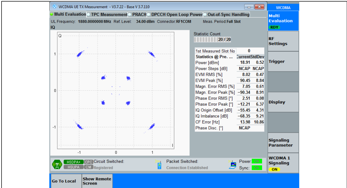
Band2_HSPA_MCH_1880MHz_Subtest 1_NTNV
