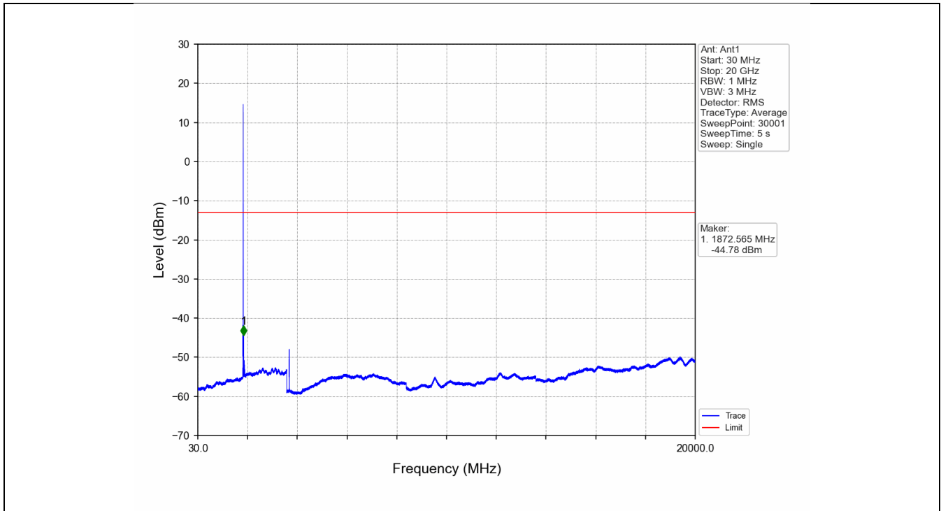
Band2_HSUPA_MCH_1880MHz_Subtest 1_NTNV
