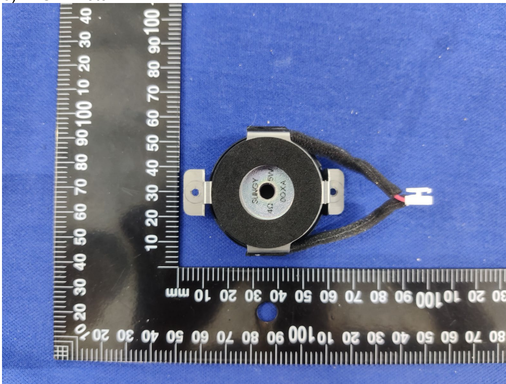
6) EUT Photo
