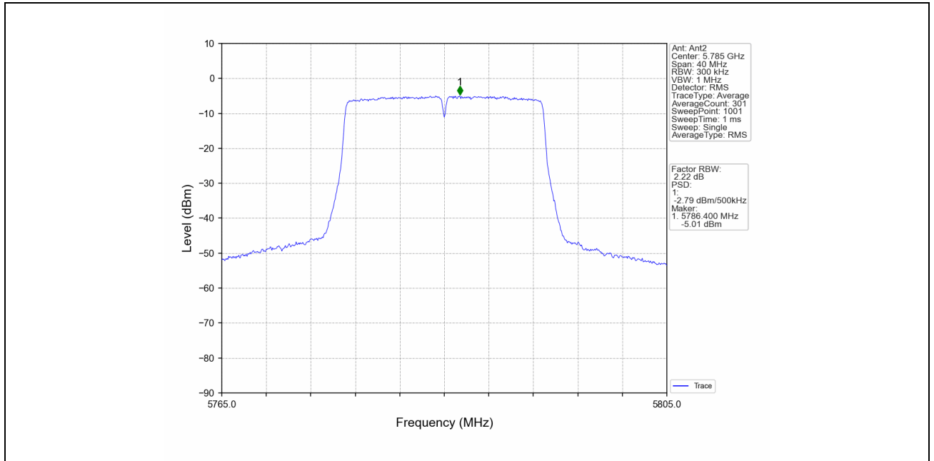
802.11n(HT20)_MCH_5785MHz_MIMO_NTNV
