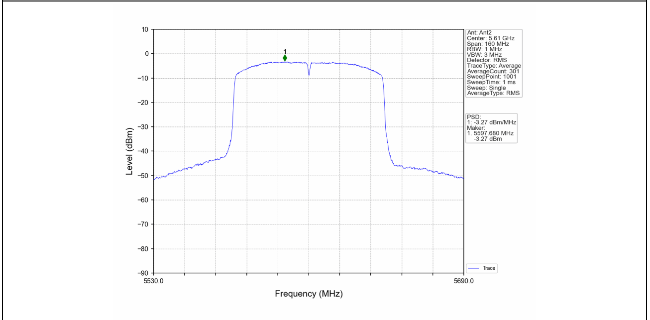
802.11ac(VHT80)_HCH_5610MHz_MIMO_NTNV
