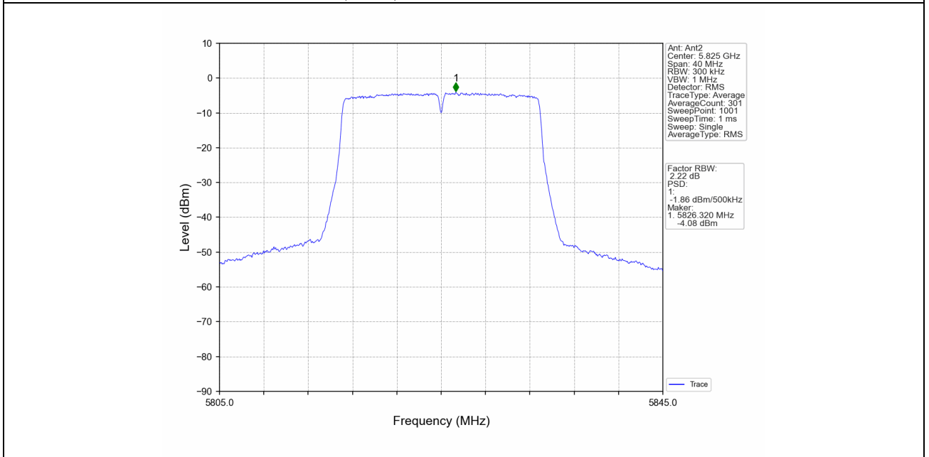
802.11n(HT20)_HCH_5825MHz_MIMO_NTNV
