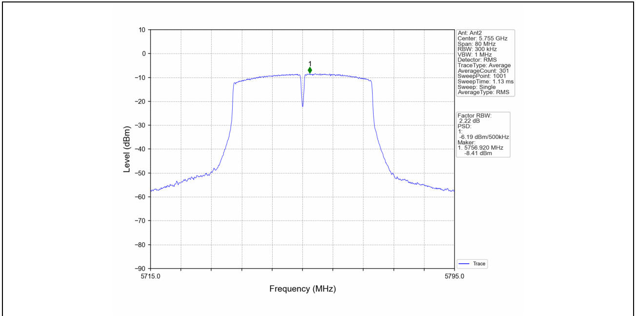
802.11n(HT40)_LCH_5755MHz_MIMO_NTNV
