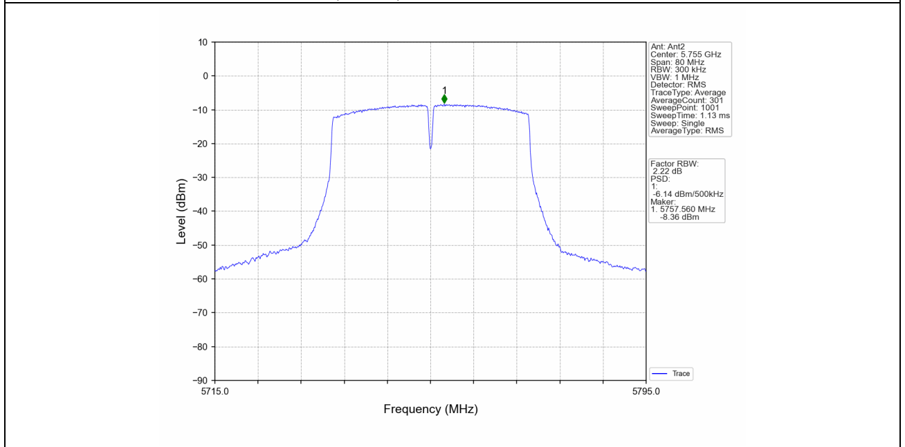
802.11ac(VHT40)_LCH_5755MHz_MIMO_NTNV
