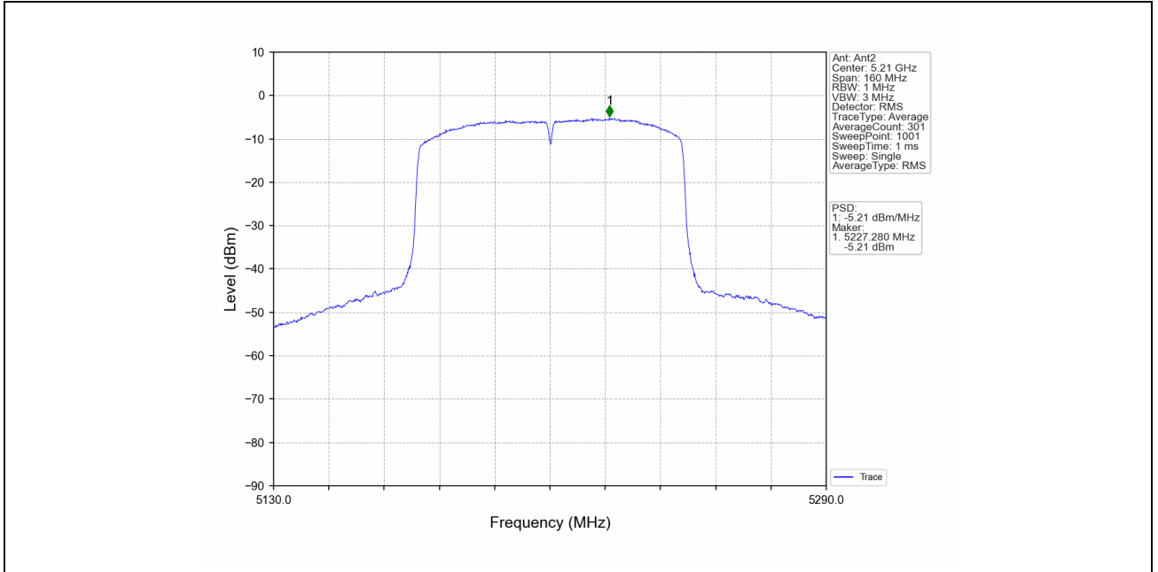
802.11ac(VHT80)_MCH_5210MHz_MIMO_NTNV
