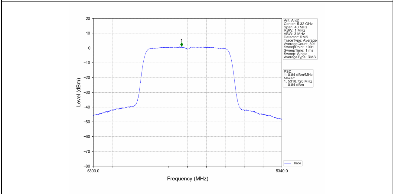
802.11n(HT20)_HCH_5320MHz_MIMO_NTNV
