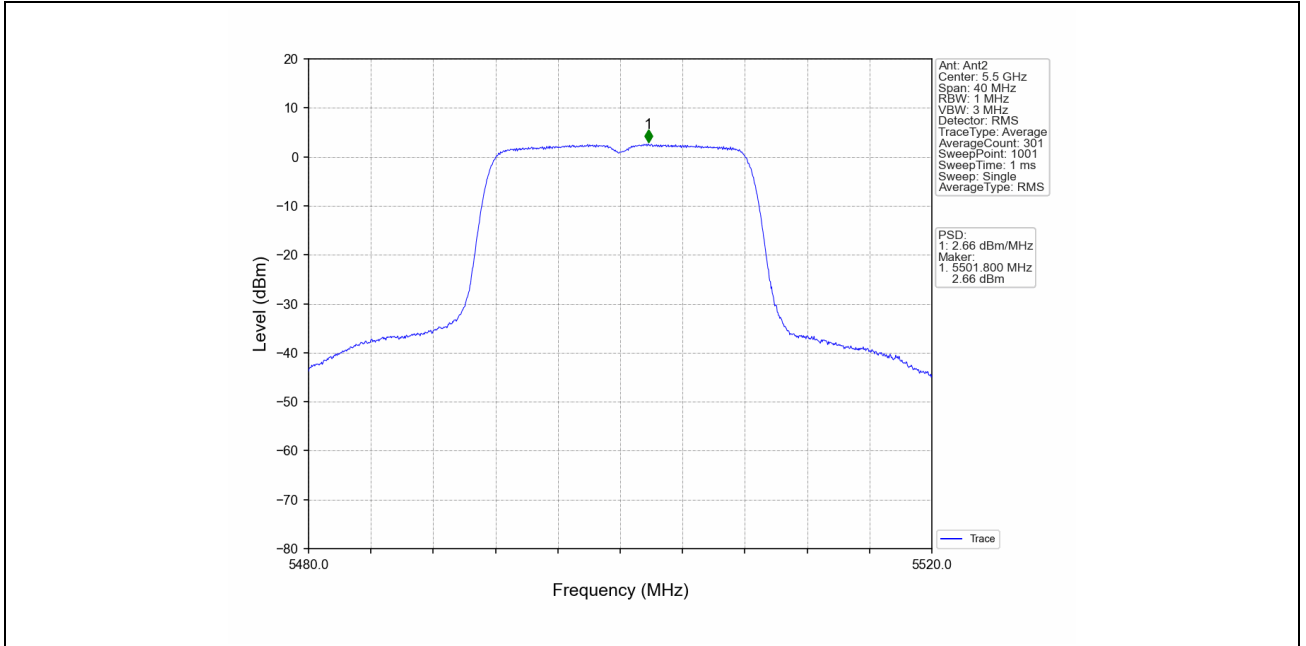
802.11n(HT20)_LCH_5500MHz_MIMO_NTNV
