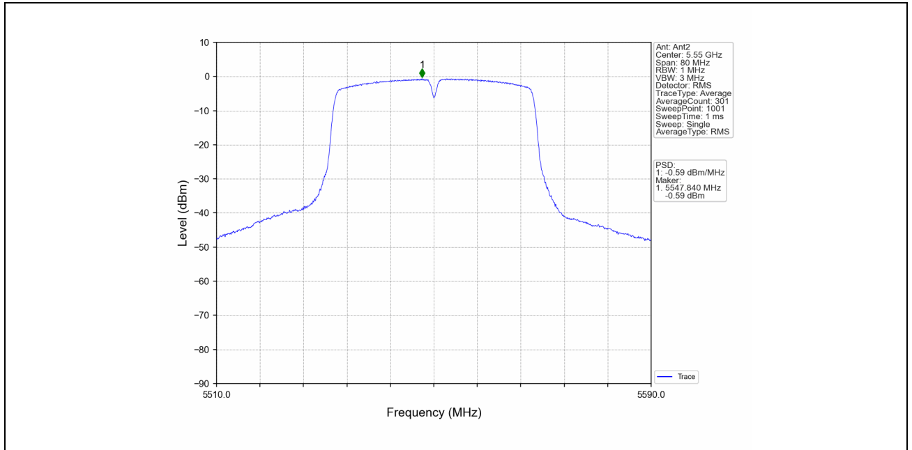
802.11n(HT40)_MCH_5550MHz_MIMO_NTNV
