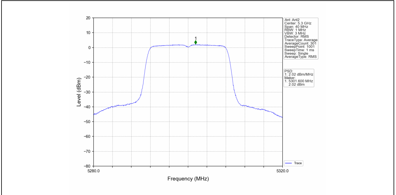
802.11n(HT20)_MCH_5300MHz_MIMO_NTNV
