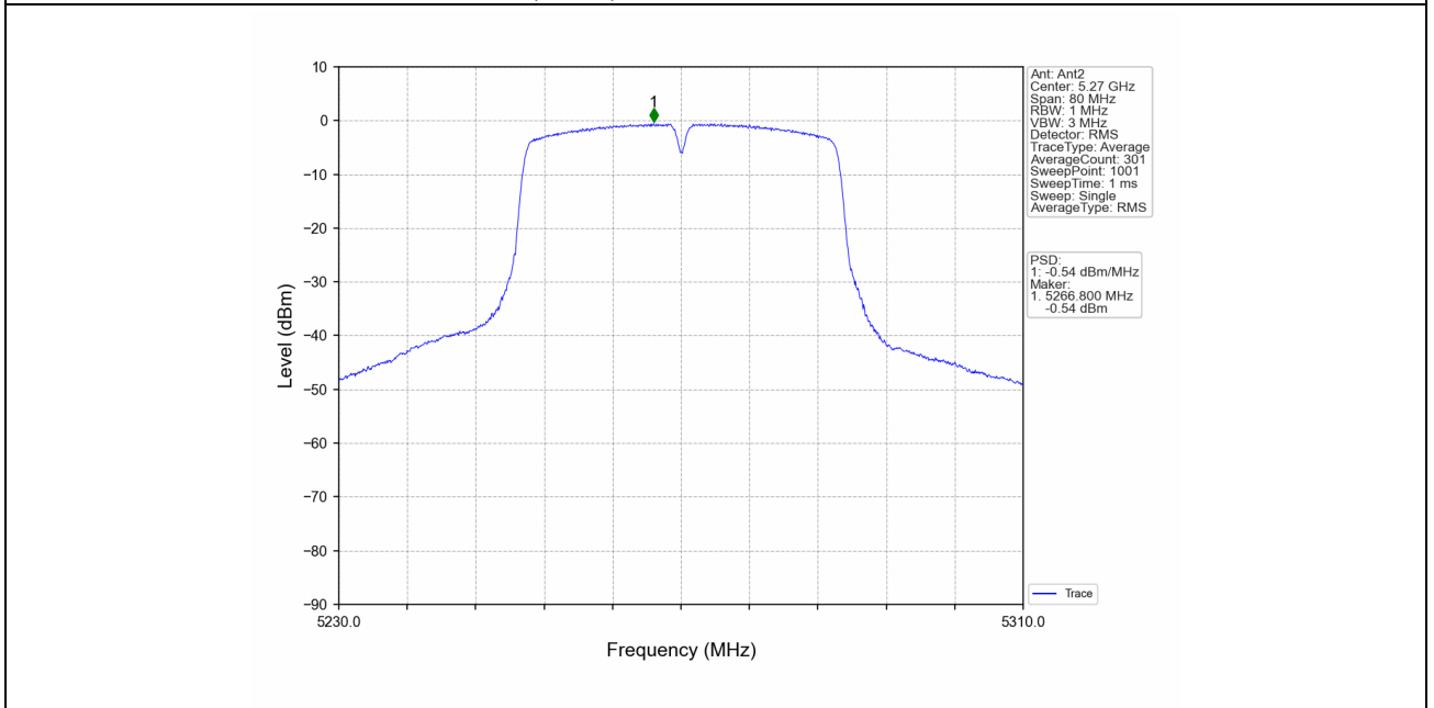
802.11n(HT40)_LCH_5270MHz_MIMO_NTNV
