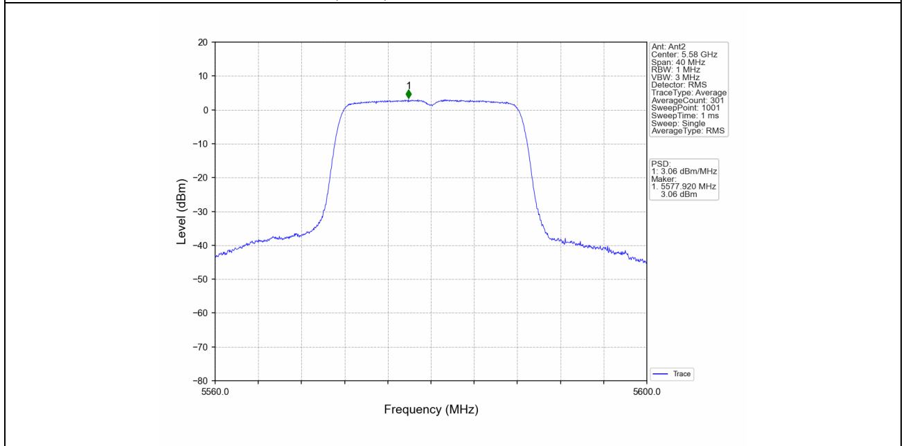
802.11n(HT20)_MCH_5580MHz_MIMO_NTNV
