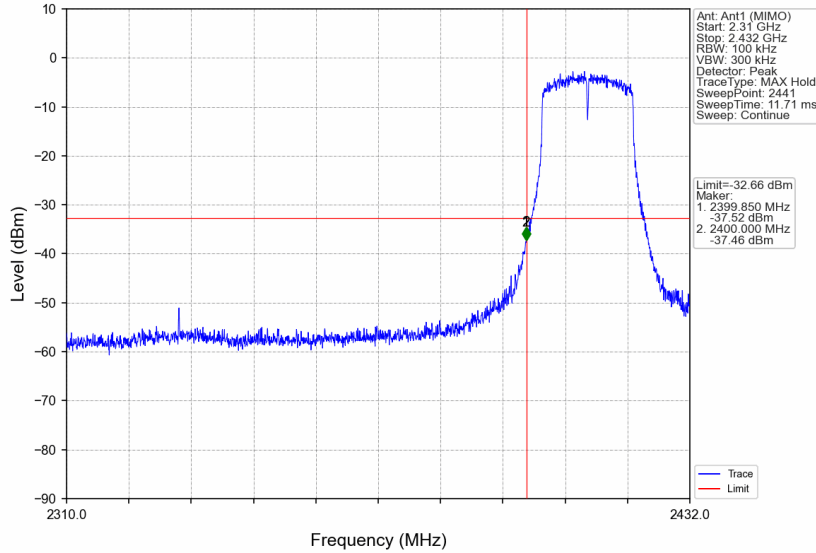
802.11n(HT20)_LCH_2412MHz_Ant1 (MIMO)_NTNV
