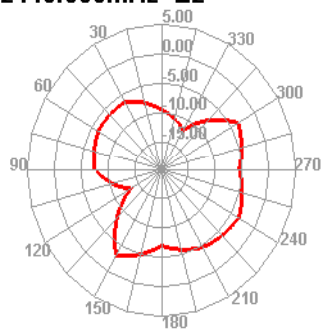
2440.000MHz E2
