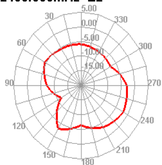
2400.000MHz E2
