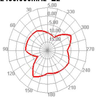
2480.000MHz E2
