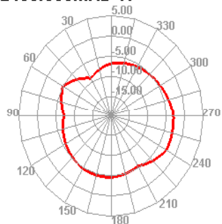
2400.000MHz H
