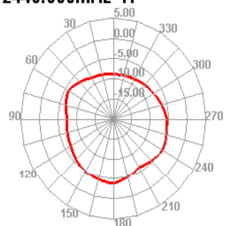
2440.000MHz H
