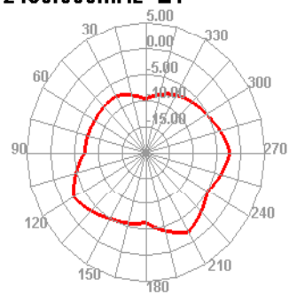
2480.000MHz E1
