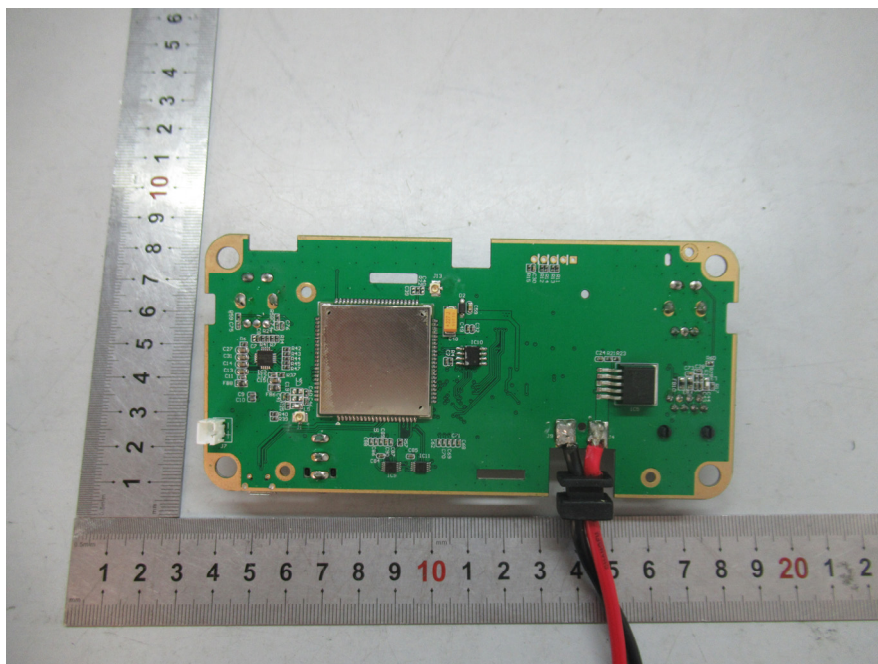
EUT(POC Mobile Radio) – PCB1 Bottom View
