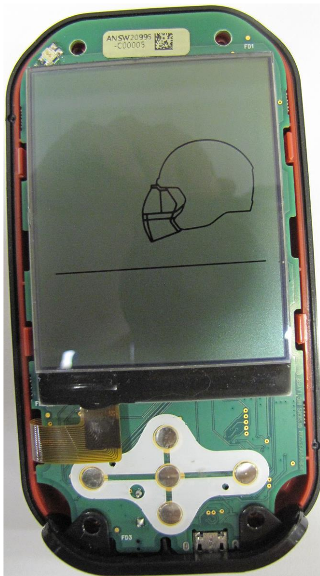
PCBA – Top side
