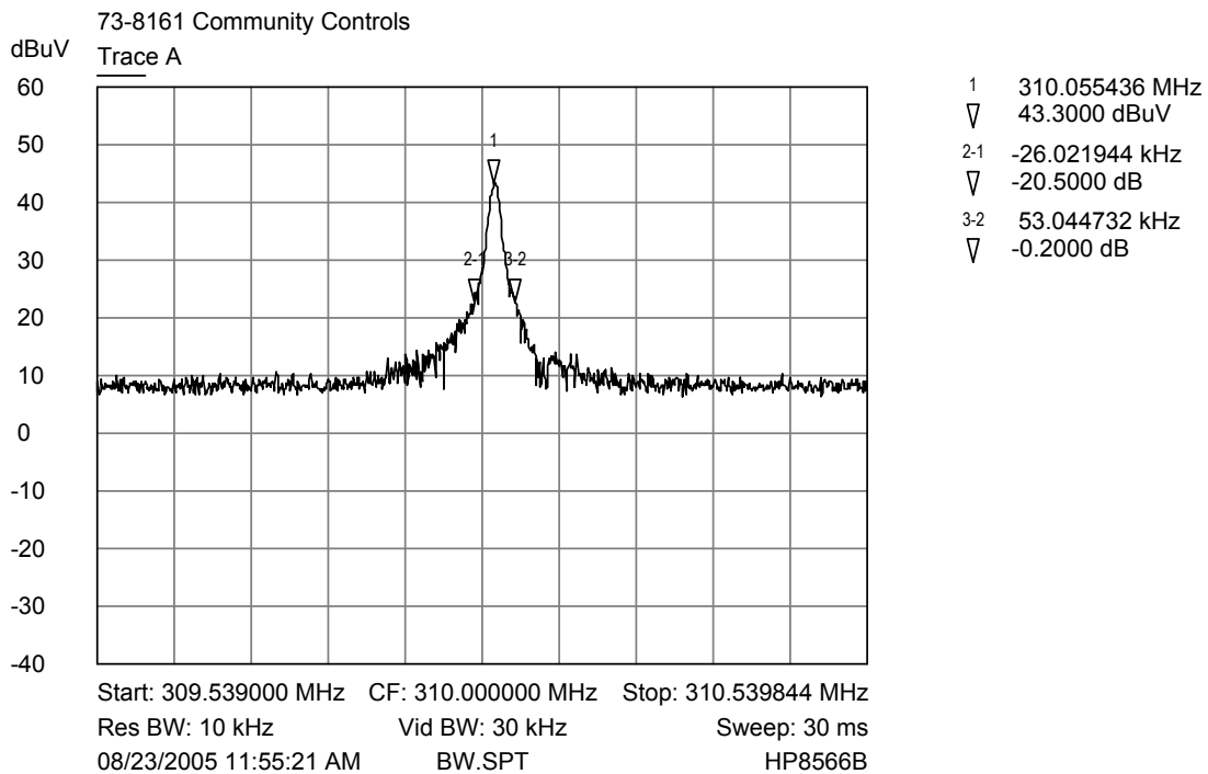
CCS3101BV Bandwidth Plot
