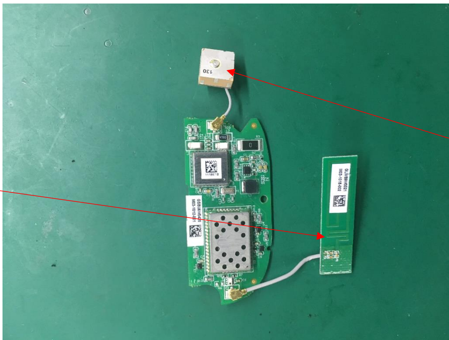
GPS Antenna
