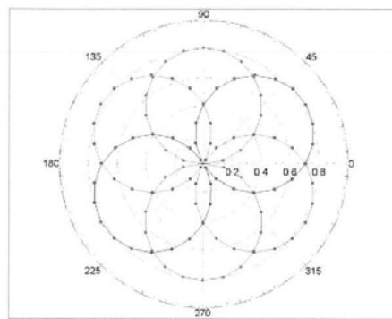
f=1800 MHz,R22
