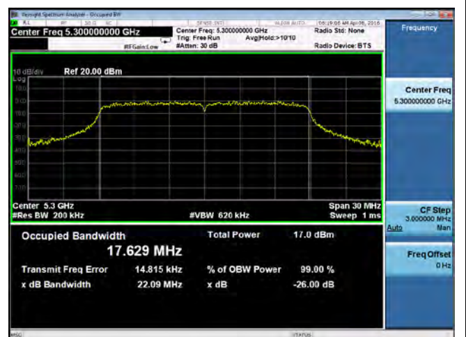
26dB BW - 802.11n-20M 5300MHz
