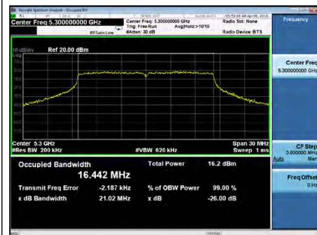
26dB BW - 802.11a 5300MHz
