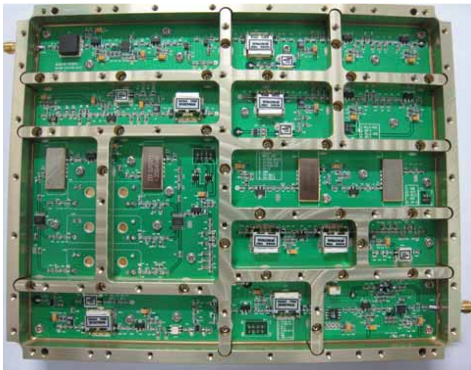
<CDMA UL Top view>
