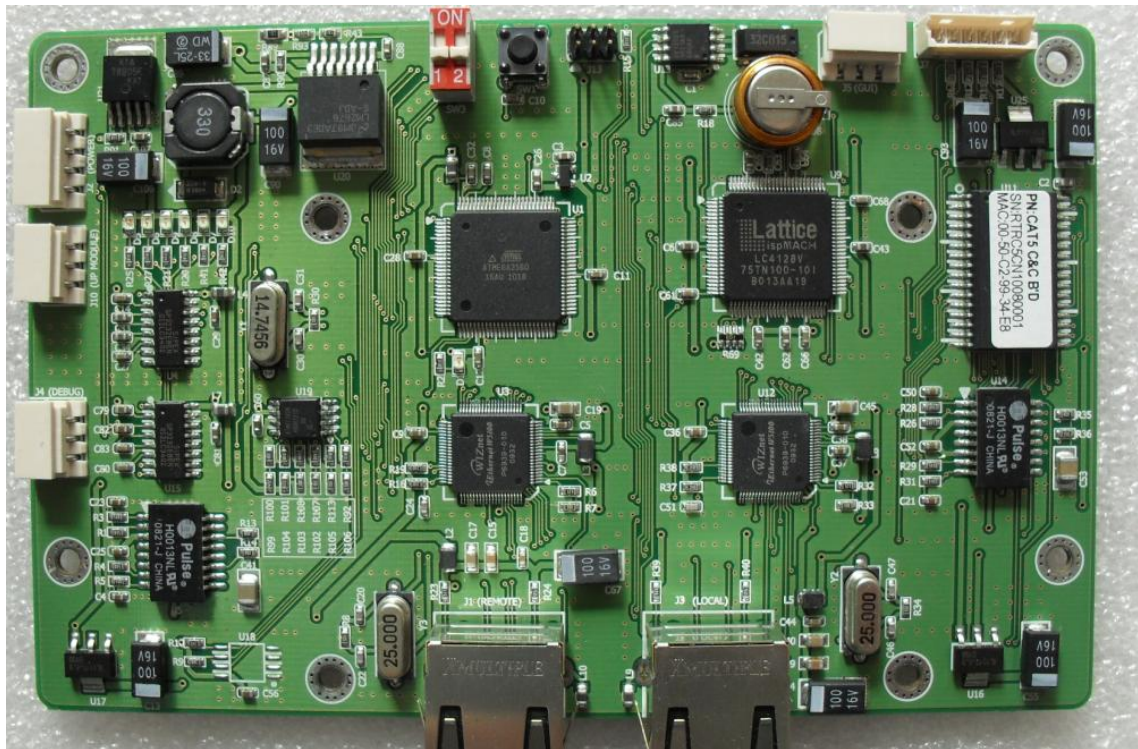
<CNC Top view>
