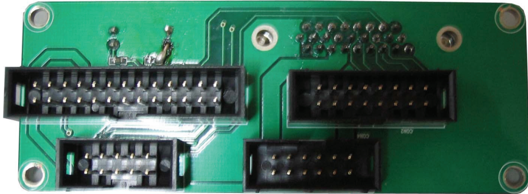
<TOP SIDE>
