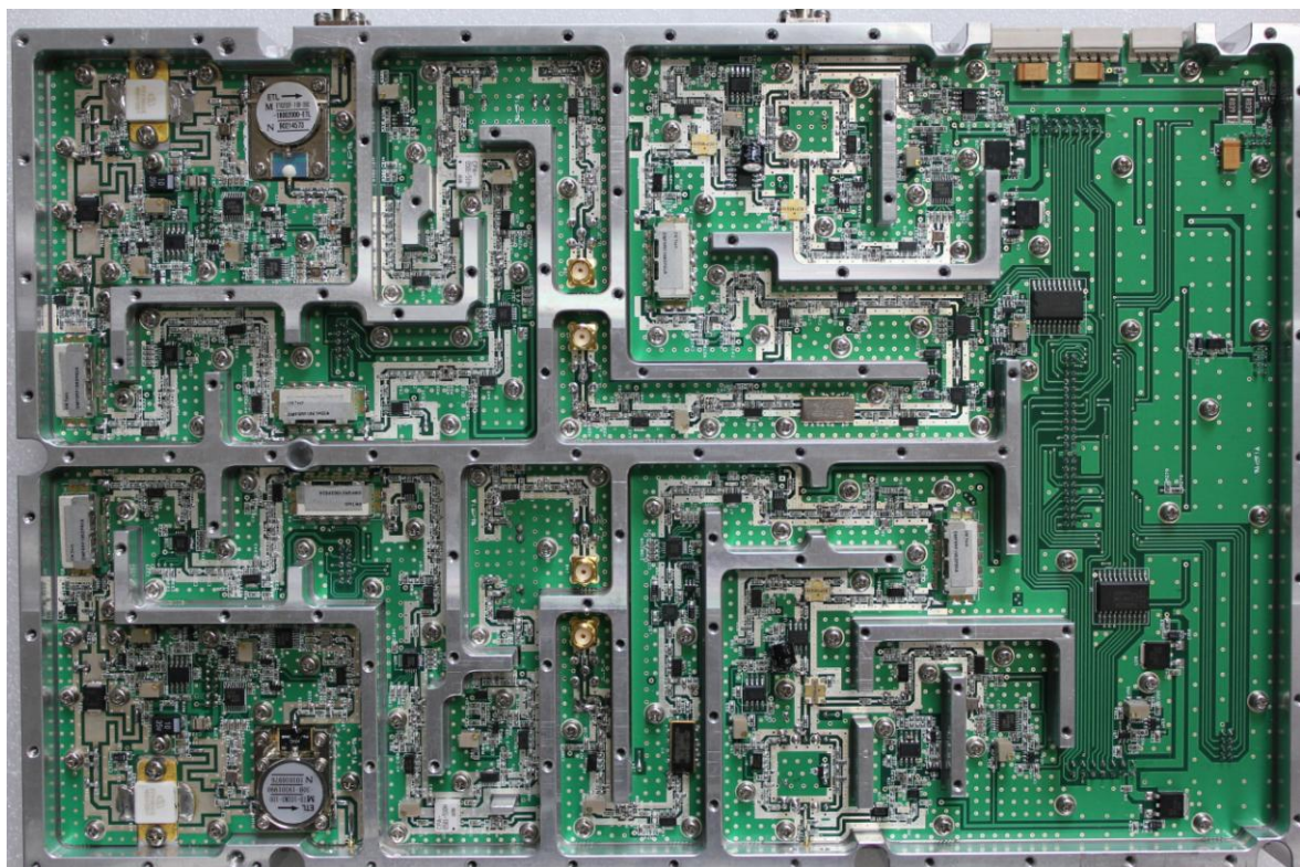
<RFU Top view>
