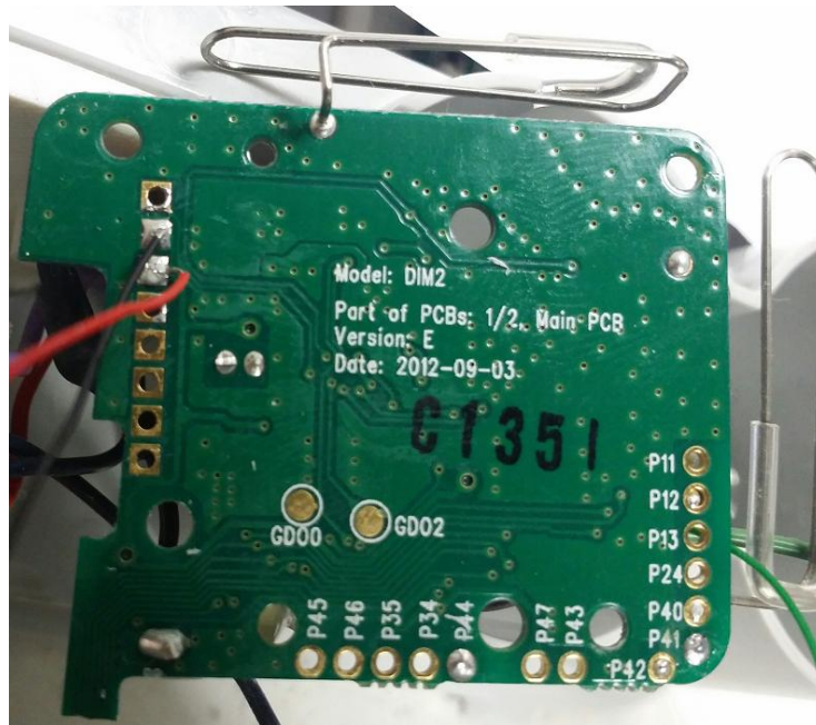
7.9 DIM 900MHz TRx PCB
