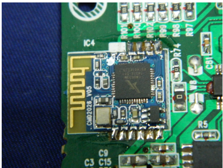
Bluetooth Module
