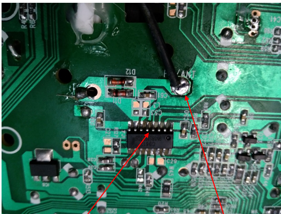
FM/AM MODULE
