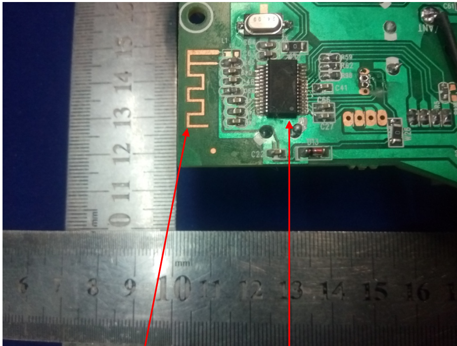
BT ATENNA
