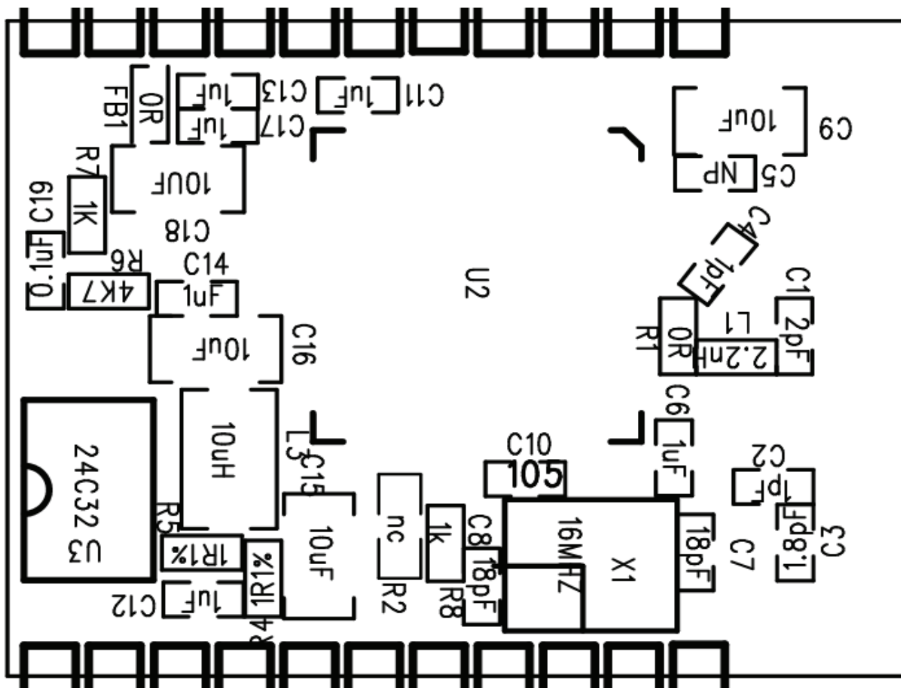
贴片图
