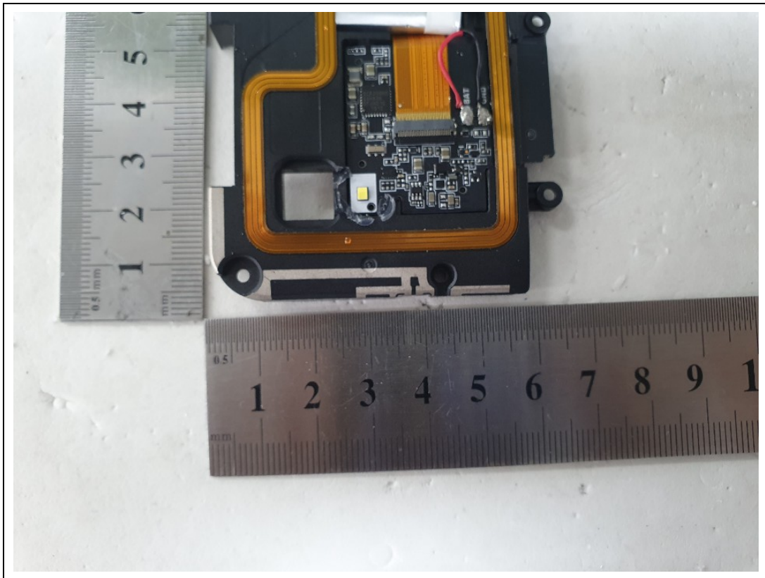
<RX Antenna>
