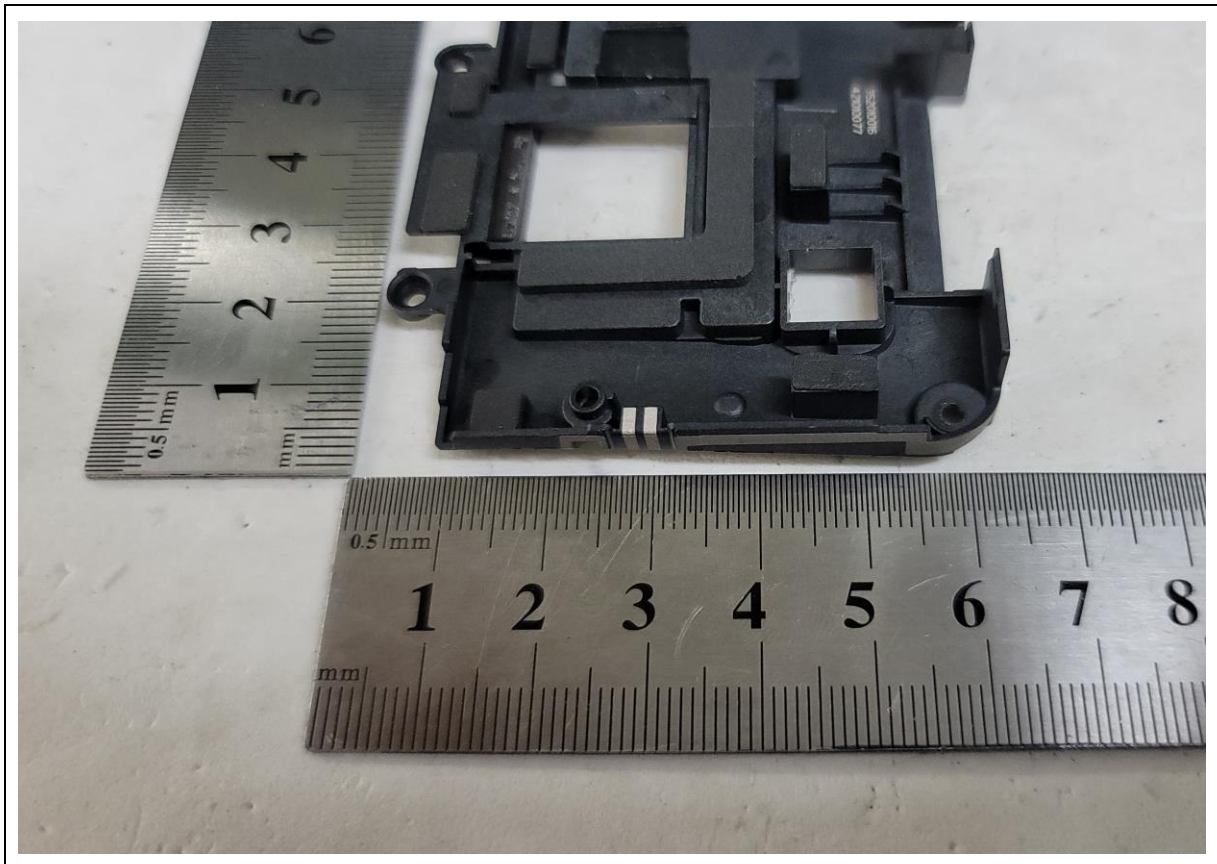
<RX Antenna>
