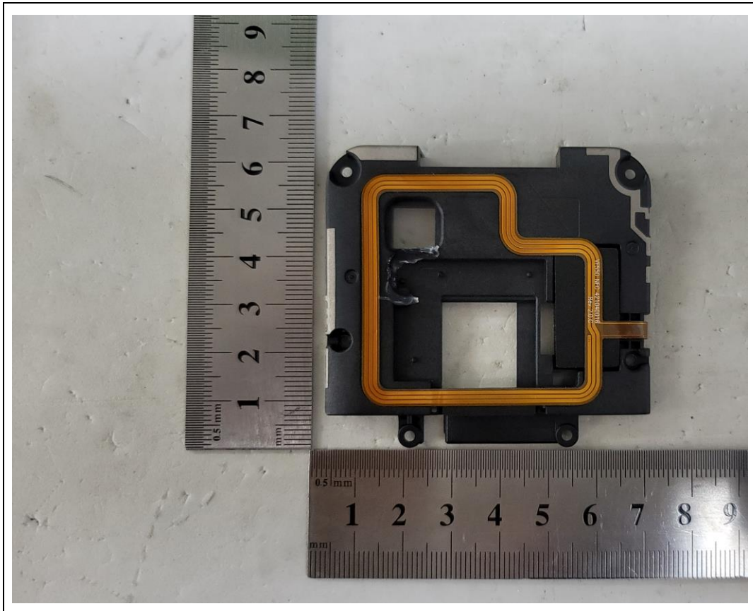
<NFC Antenna>
