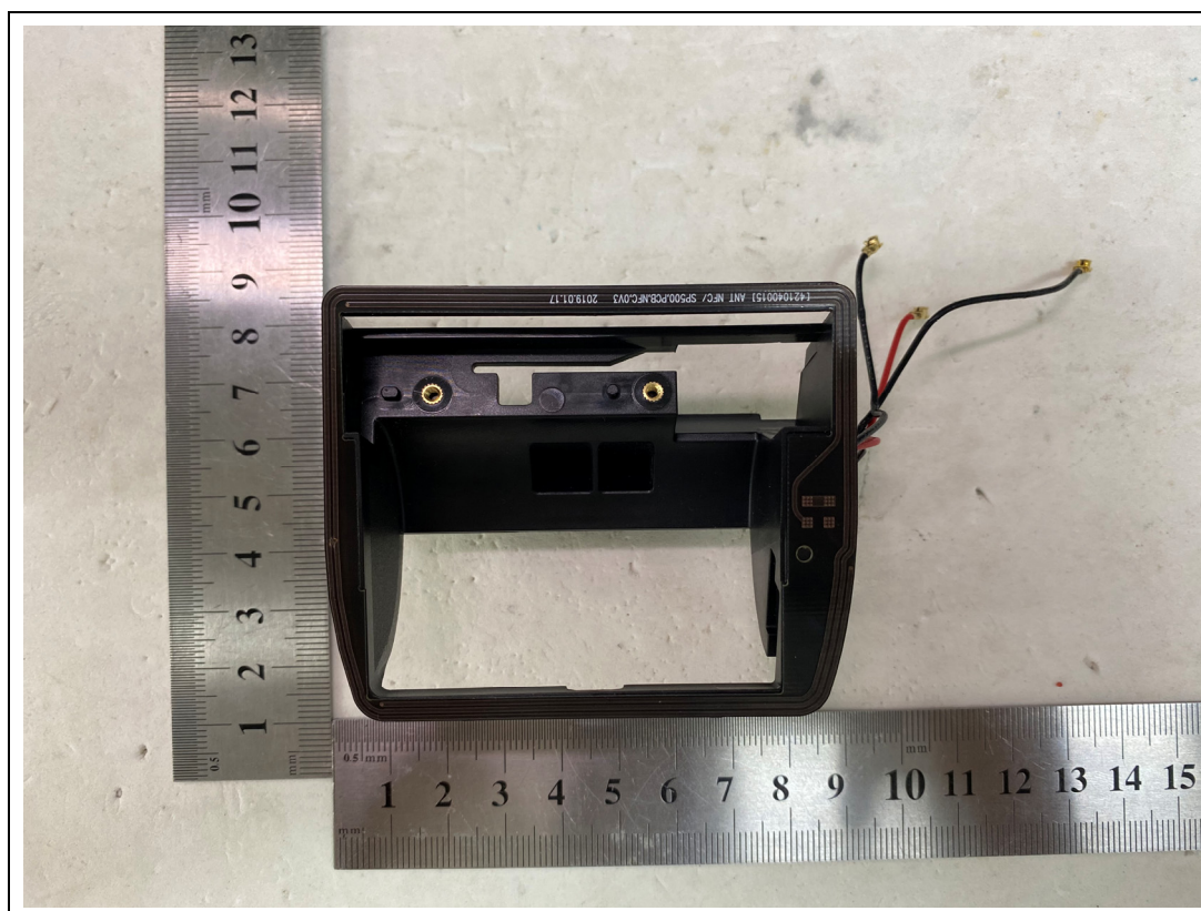
<NFC Antenna>
