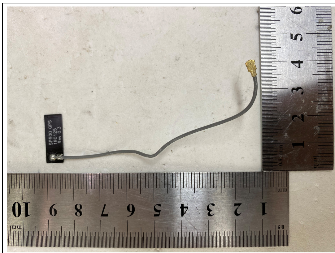
<GPS Antenna>
