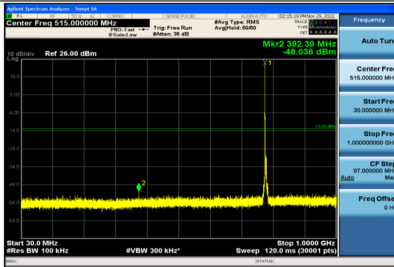
Band13-5MHz-QPSK-23230-1RB#0-30~1000MHz
