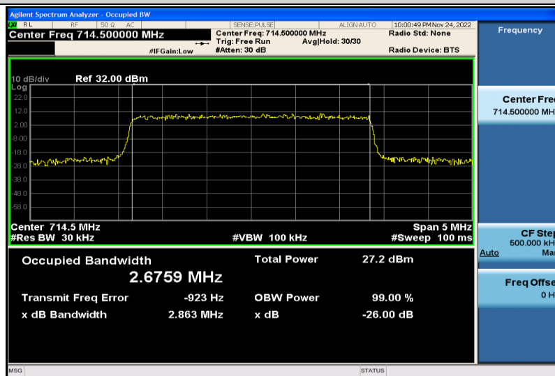
Band12-3MHz-QPSK-23165-15RB#0-2.6759
