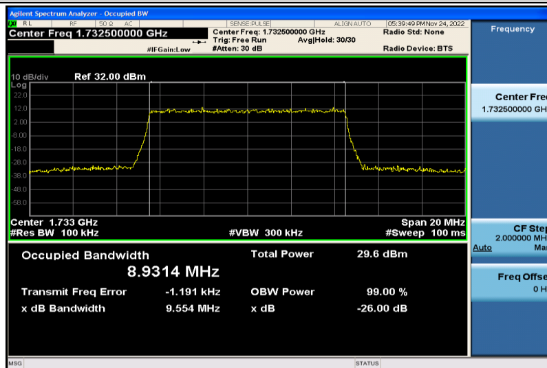
Band4-10MHz-QPSK-20175-50RB#0-8.9314
