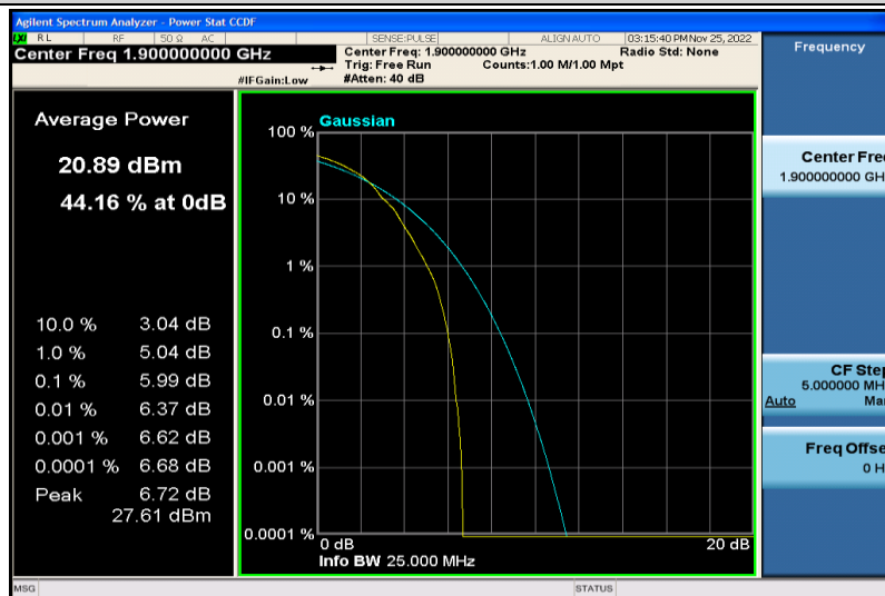
Band2-20MHz-64QAM-19100-1RB#0
