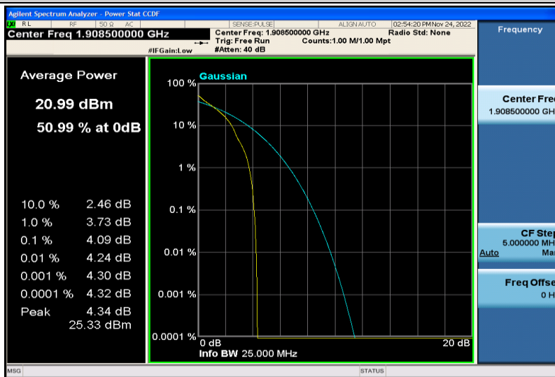
Band2-3MHz-QPSK-19185-1RB#0
