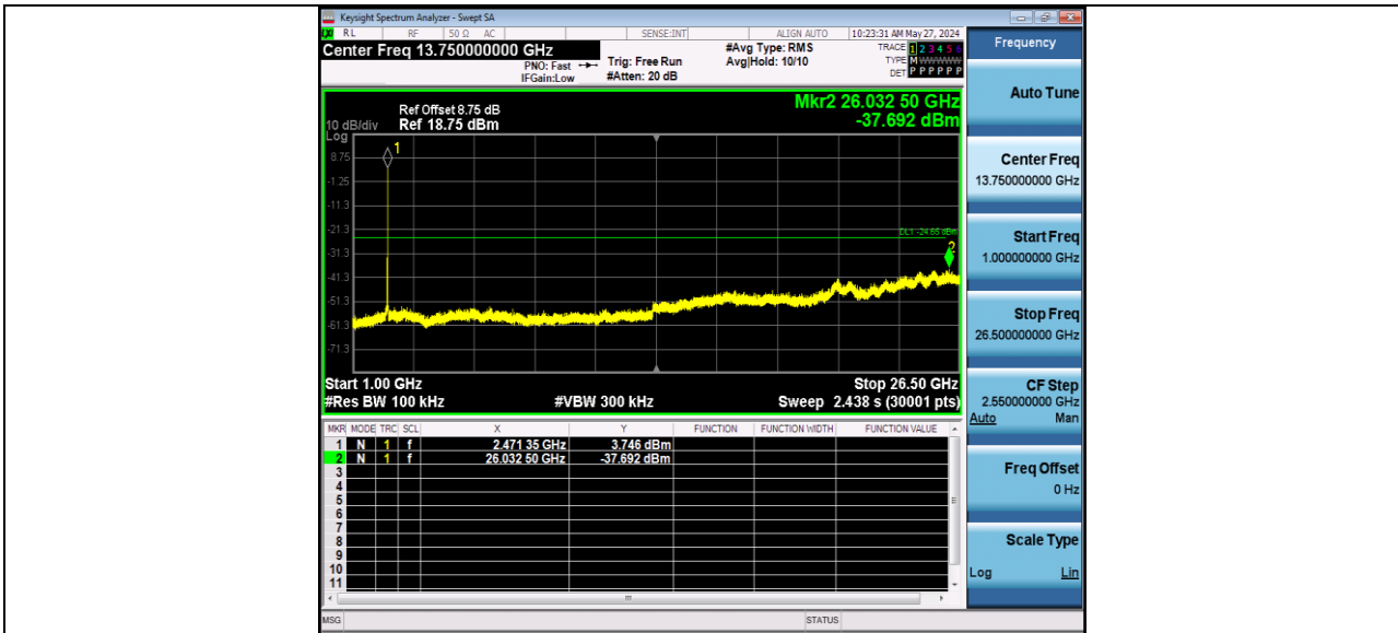
11AX20MIMO_Ant2_2462_106Tone_RU54_0~Reference
