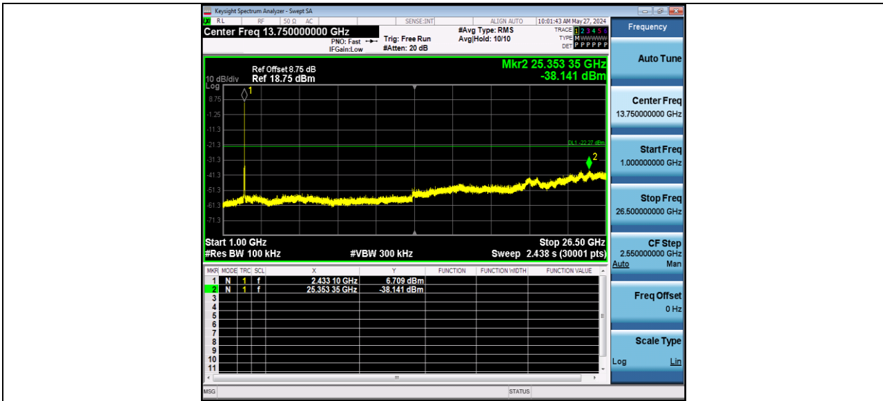
11AX20MIMO_Ant2_2437_106Tone_RU53_0~Reference
