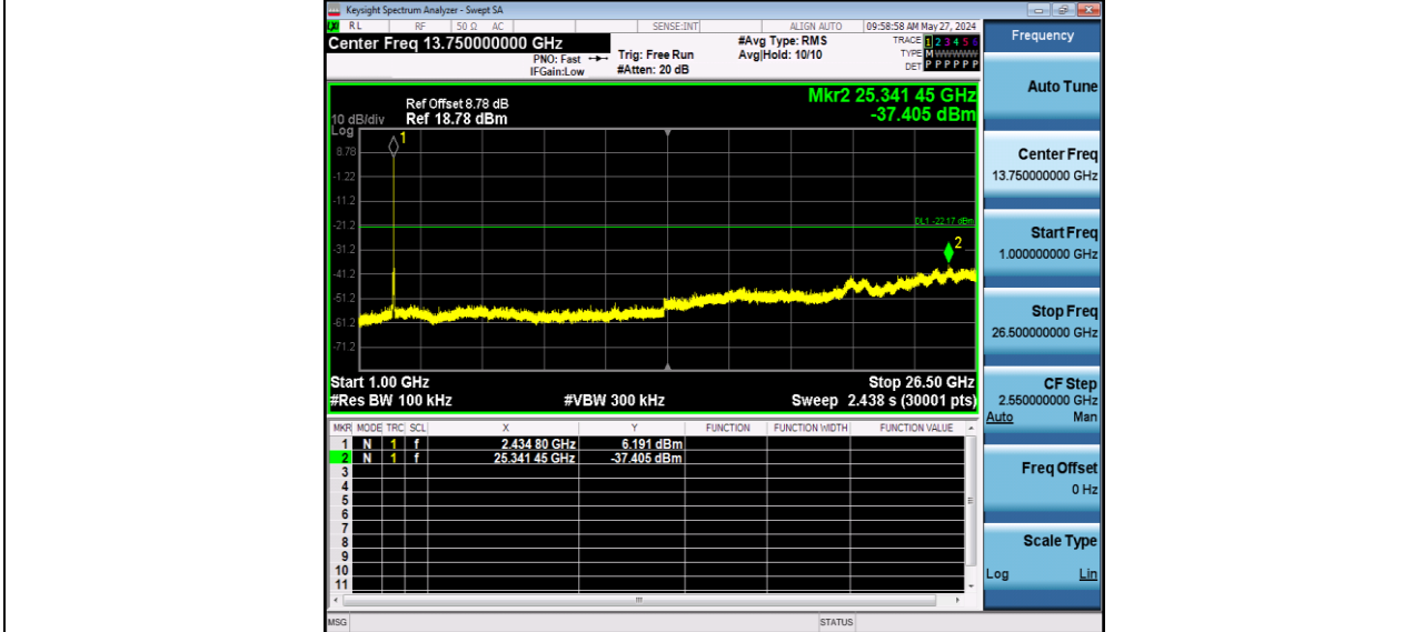
11AX20MIMO_Ant1_2437_106Tone_RU53_0~Reference
