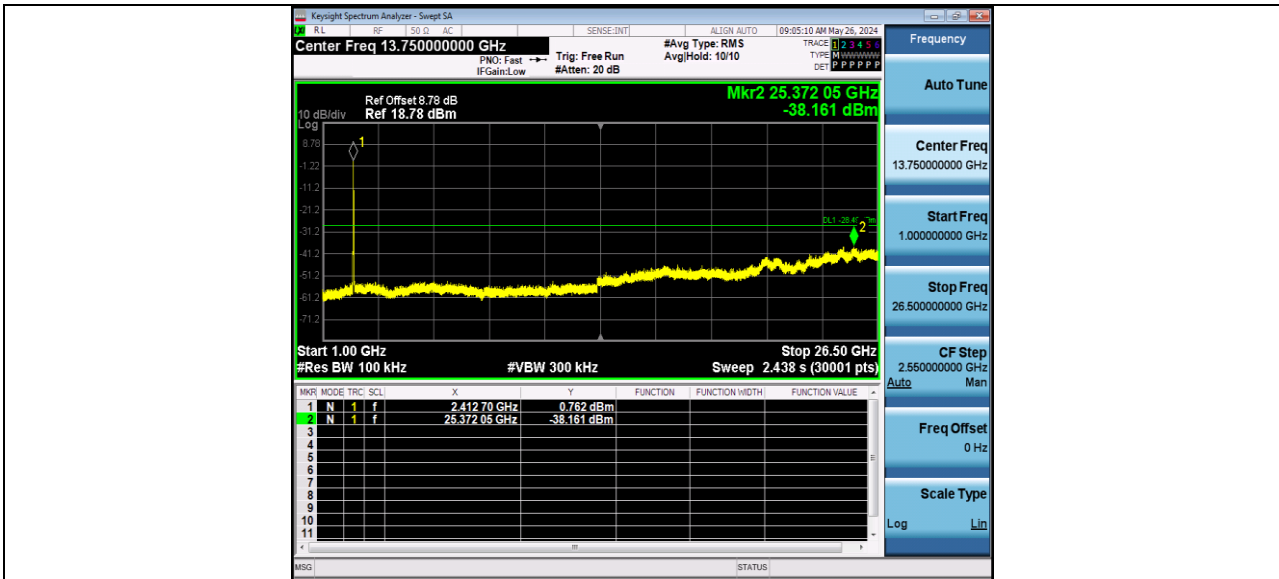
11AX20MIMO_Ant2_2412_0-Reference
