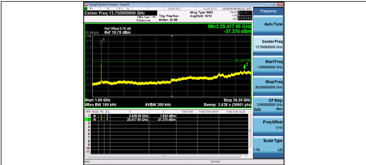
11AX20MIMO Ant2_2437_0-Reference
