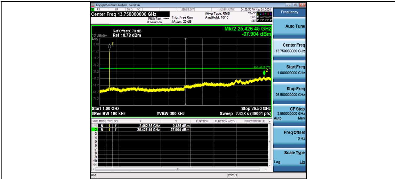
11N/AC 20MIMO_Ant2_2462_0-Reference
