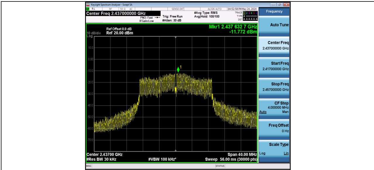
11N/AC 20MIMO_Ant2_2437
