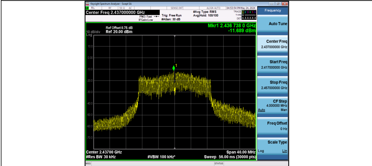
11N/AC 20MIMO_Ant1_2462
