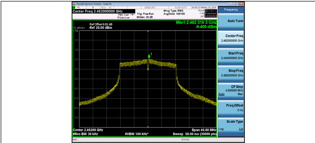
11G-CDD_Ant2_2462
