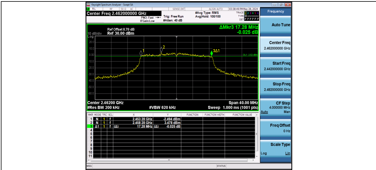
11N/AC 20MIMO_Ant2_2462
