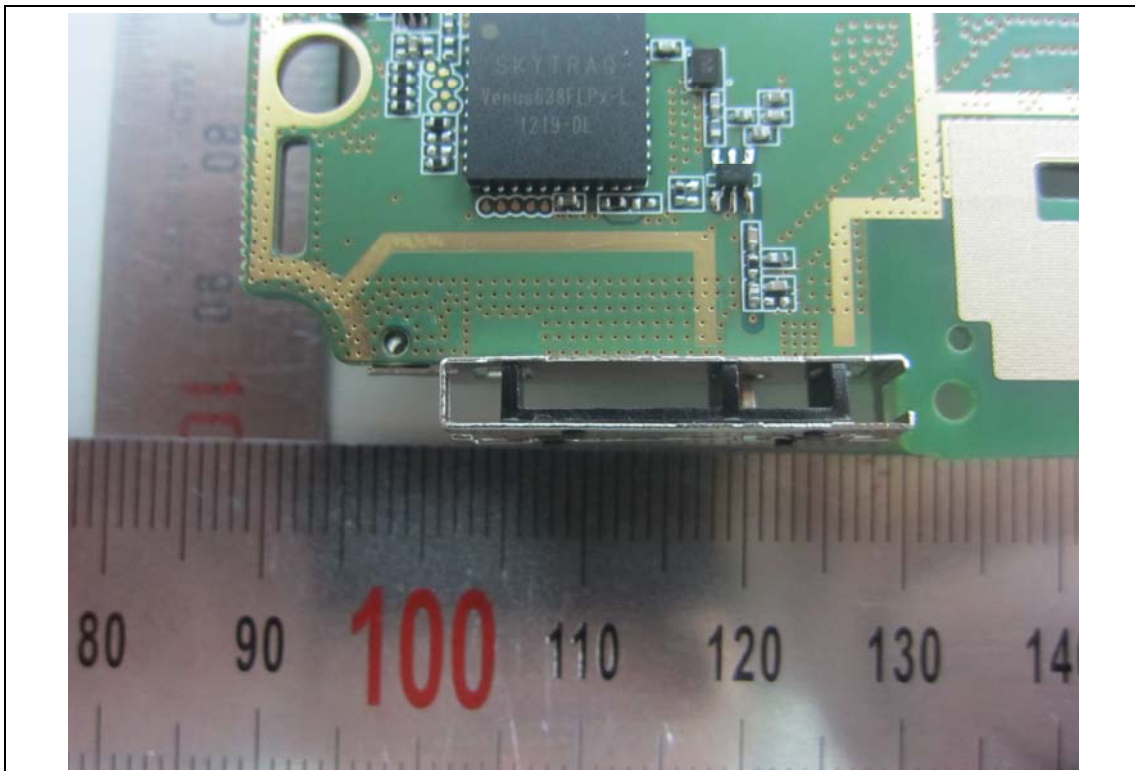
GPS Antenna
