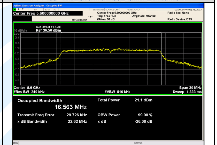
IEEE 802.11a Channel 120_20MHz Antenna 1
