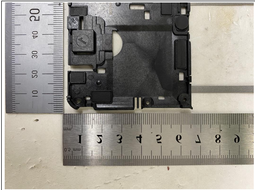
<RX Antenna>
