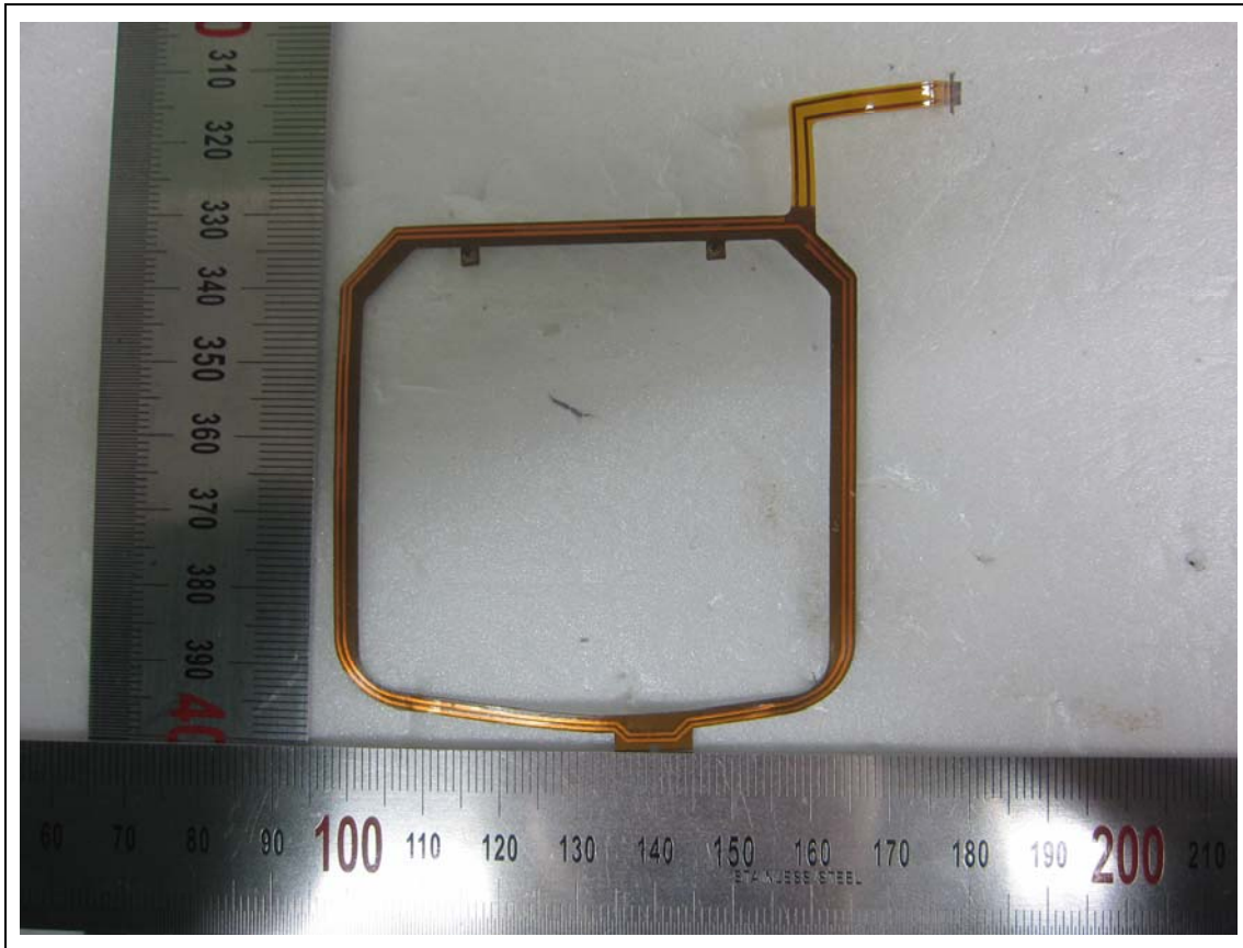
-RFID Ant-
