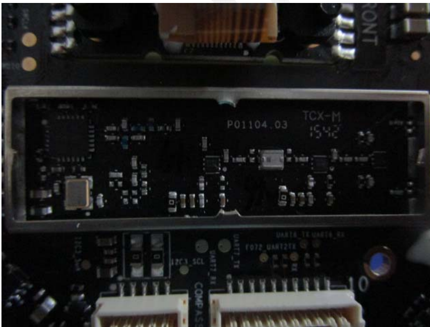
EUT –5.8G Module View
