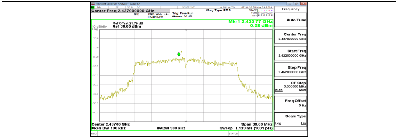
11N20MIMO_Ant3_2437_0~Reference
