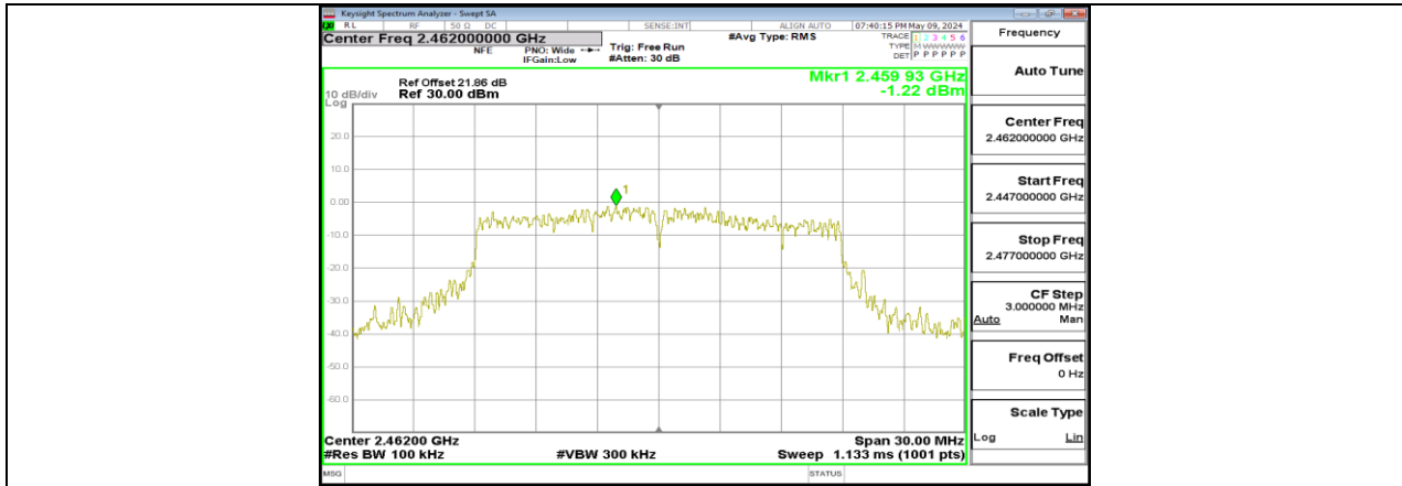
11N20MIMO_Ant3_2462_0~Reference
