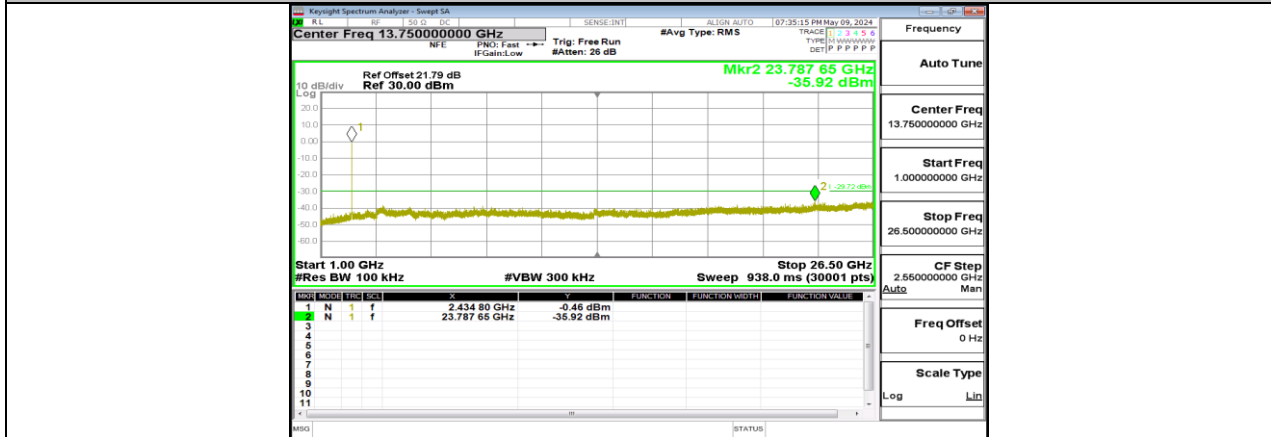
11N20MIMO_Ant3_2437_1000~26500
