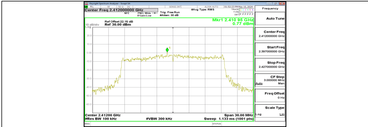
11AX20MIMO_Ant3_2412_0-Reference
