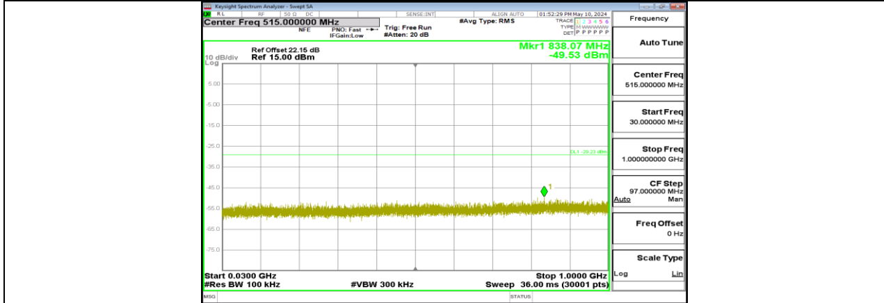
11AX20MIMO_Ant3_2412_30-1000
