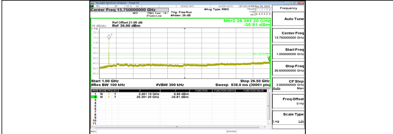
11B_Ant3_2462_1000~26500
