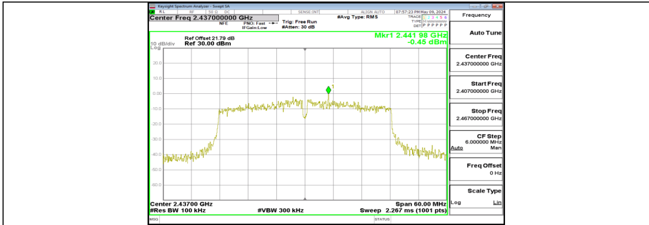
11N40MIMO_Ant3_2437_0~Reference
