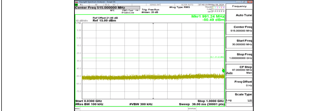
11N20MIMO_Ant3_2462_30~1000
