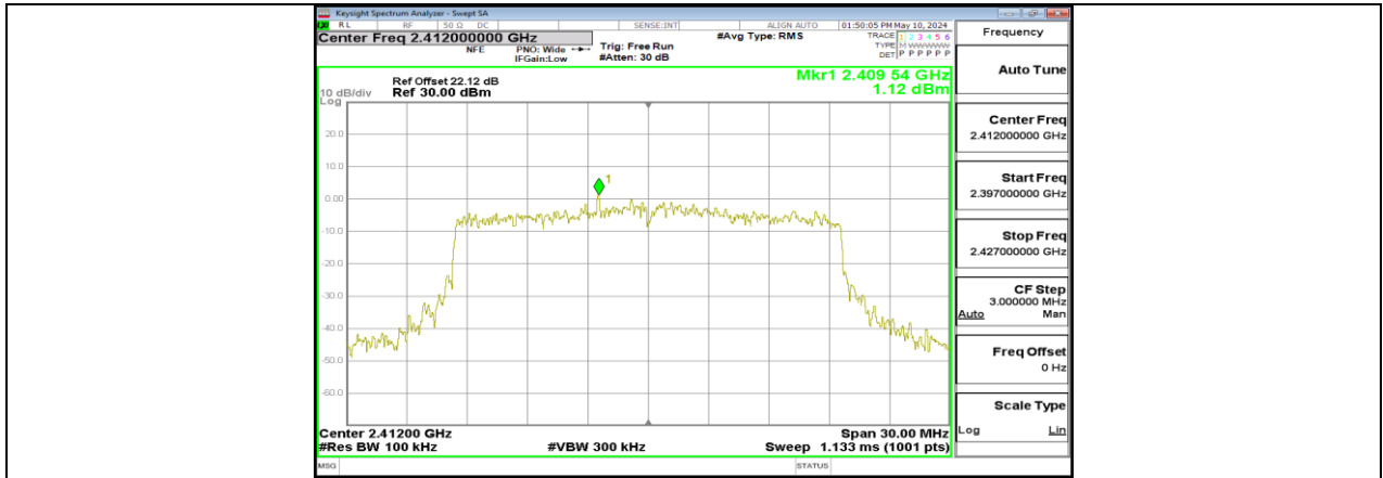
11AX20MIMO_Ant2_2412_0-Reference
