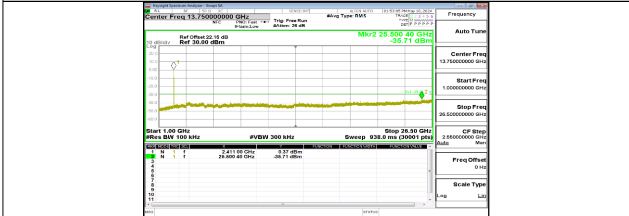
11AX20MIMO_Ant3_2412_1000-26500
