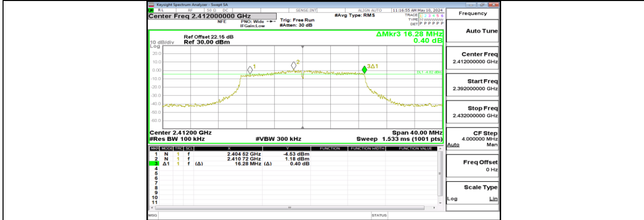
11N20MIMO_Ant3_2412
