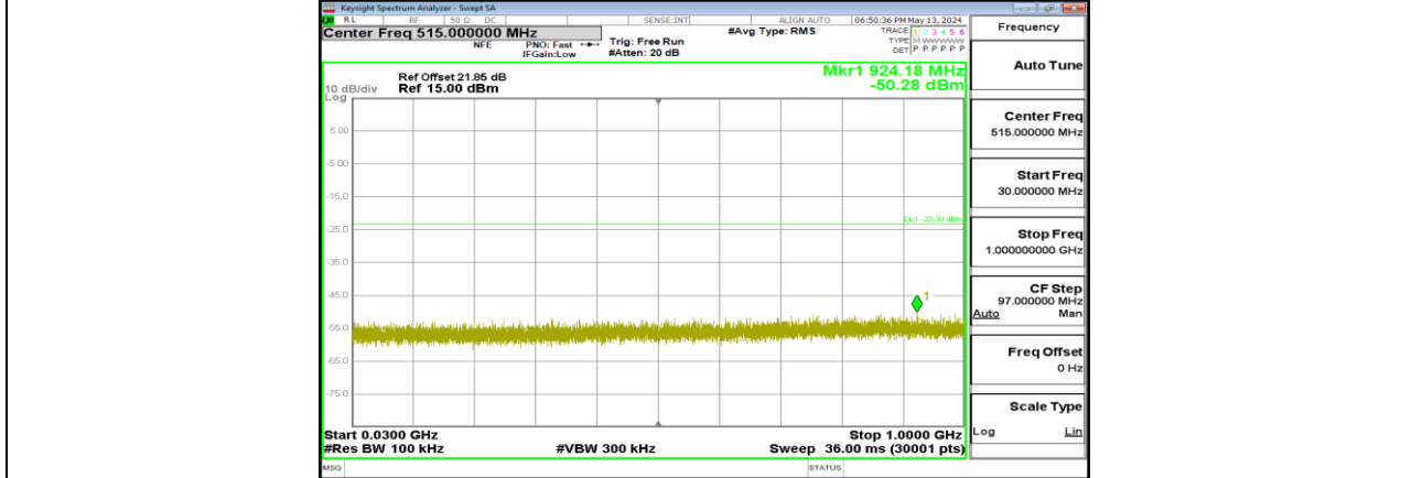
3DH5_Ant2_2480_30~1000
