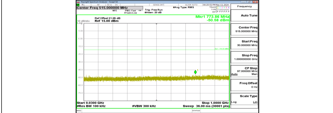
DH5_Ant2_2480_30-1000
