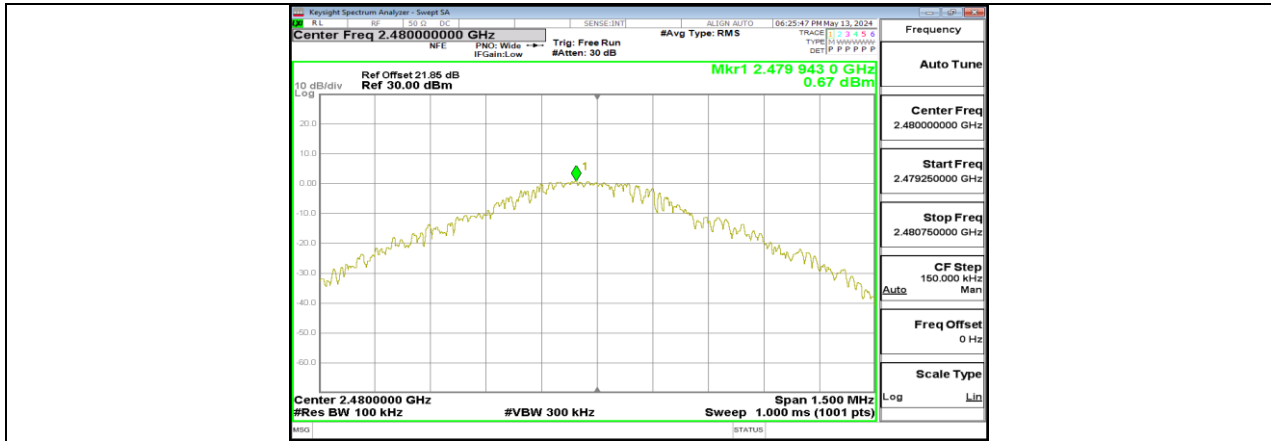
DH5_Ant2_2480_0-Reference
