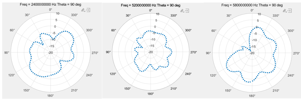
Ant 1 (左外置全向天线)
