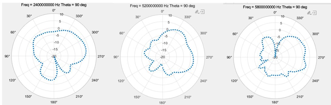
Ant 0 (右外置全向天线)
