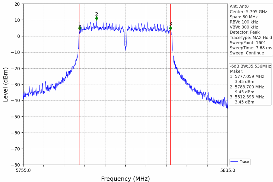
802.11n(HT40)_HCH_5795MHz_Ant0_NTNV
