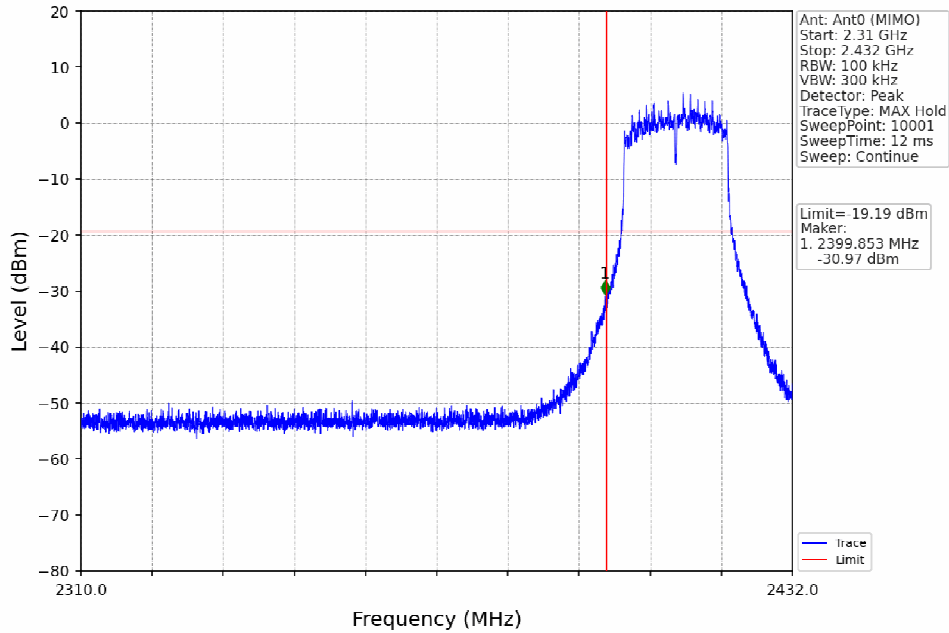
802.11n(HT20)_LCH_2412MHz_Ant0 (MIMO)_NTNV
