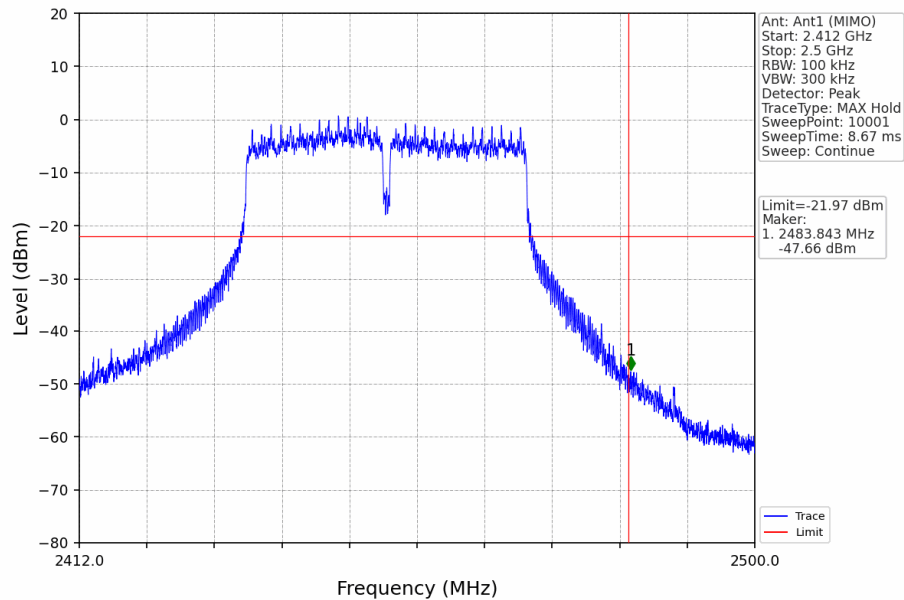
802.11n(HT40)_HCH_2452MHz_Ant1 (MIMO)_NTNV
