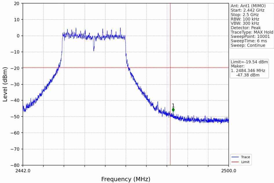
802.11n(HT20)_HCH_2462MHz_Ant1 (MIMO)_NTNV
