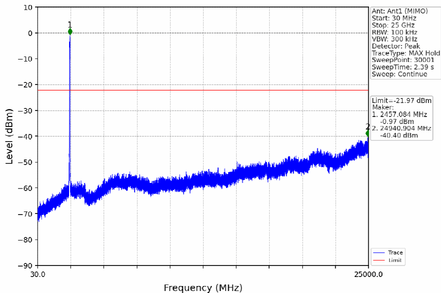
802.11n(HT40)_HCH_2452MHz_Ant1 (MIMO)_NTNV
