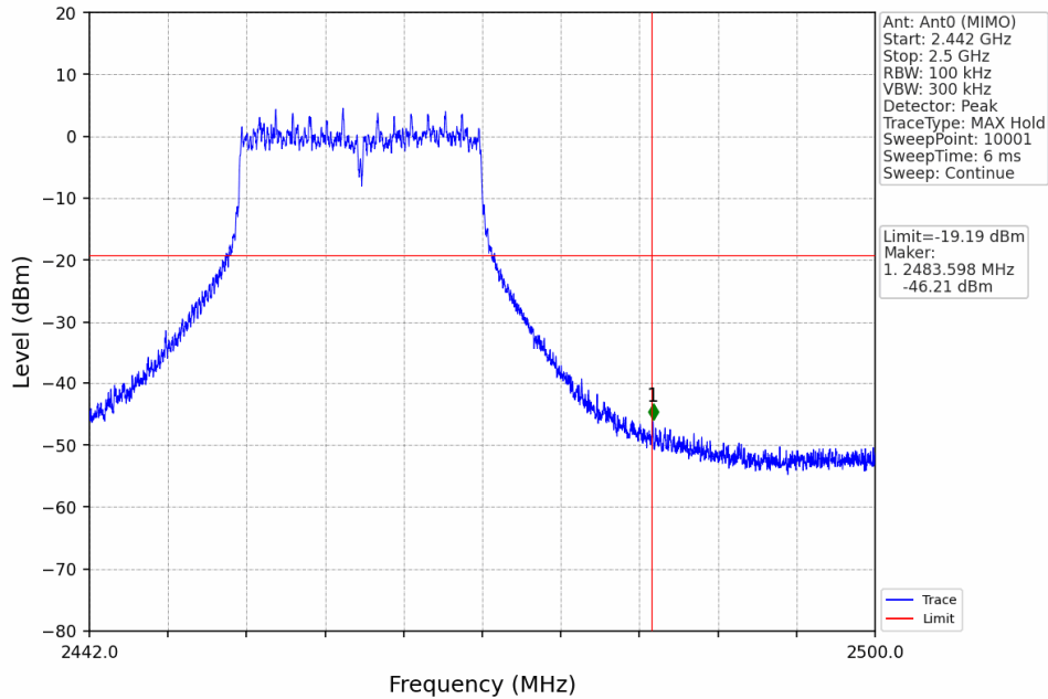
802.11n(HT20)_HCH_2462MHz_Ant0 (MIMO)_NTNV
