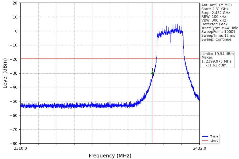
802.11n(HT20)_LCH_2412MHz_Ant1 (MIMO)_NTNV
