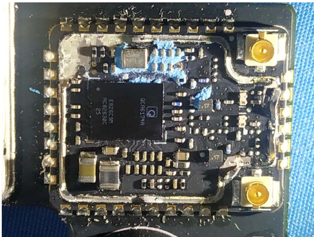
SDR Module
